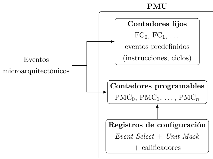
Figura 0.2: Organización conceptual de una Unidad de Monitorización de Rendimiento (PMU) con contadores fijos y programables. Elaboración propia.
