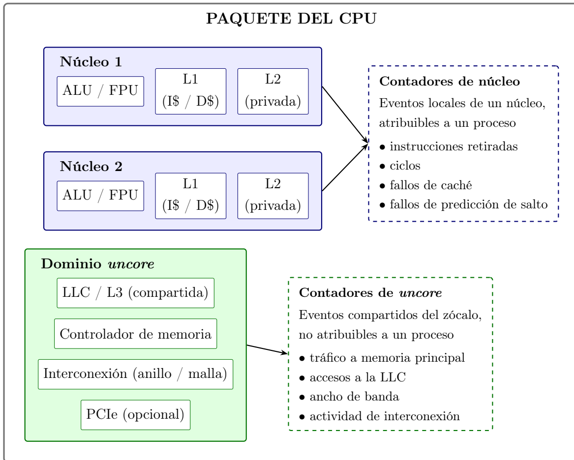
Figura 0.3: Ámbito de atribución de los contadores de núcleo y de uncore dentro del paquete del procesador. Los contadores de núcleo observan eventos locales de un núcleo concreto y pueden asociarse a un proceso; los de uncore observan recursos compartidos del zócalo y son de alcance de sistema. Elaboración propia.
