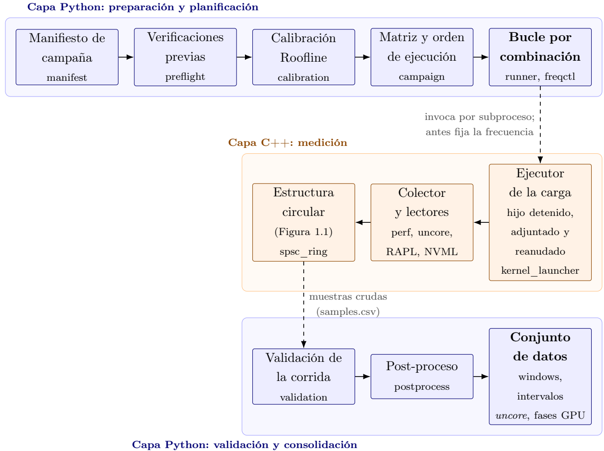
Figura 1.2: Recorrido de una campaña a través de las dos capas del instrumento. La capa Python prepara la campaña (banda superior), invoca por subproceso el ejecutor de la capa C++ una vez por combinación de carga y frecuencia (banda intermedia), y consolida las muestras crudas que este produce en el conjunto de datos (banda inferior). La capa C++ concentra la medición sensible a la latencia y la capa Python administra la lógica experimental.
