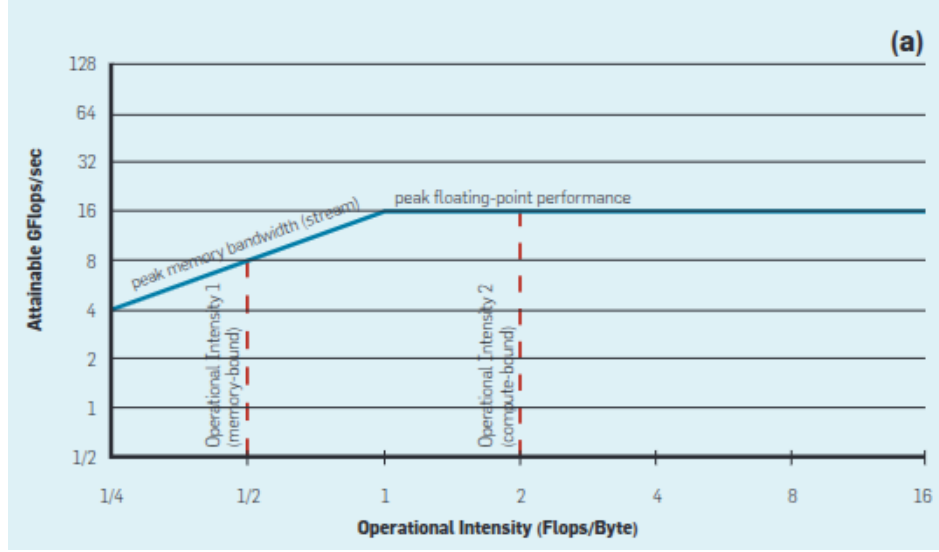
Figura 0.1: Modelo Roofline conceptual de la relación entre el techo de ancho de banda de memoria y el techo de rendimiento de cómputo. Tomado de Williams et al. [46, Fig. 1(a)].
