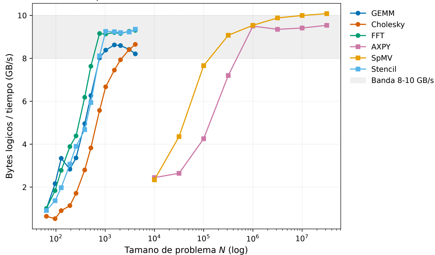
Rendimiento implícito de movimiento de datos, GPU en caliente (REF)
