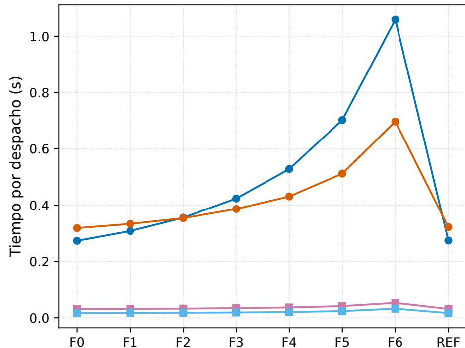
CPU (cpu:F0..F6,REF)
