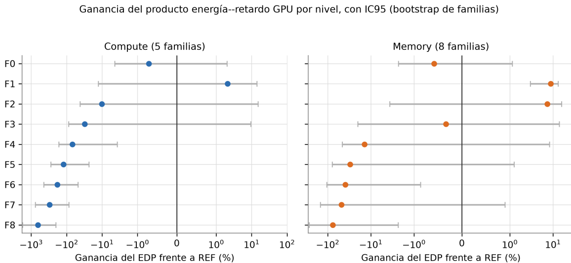
Figura 3.25: Misma información de la Tabla 3.20, en forma gráfica, con la familia como unidad. El eje horizontal es simétrico-logarítmico para mostrar a la vez F1, cercano a cero, y F8, con pérdidas de más de un orden de magnitud en compute_bound . Fuente: elaboración propia.
