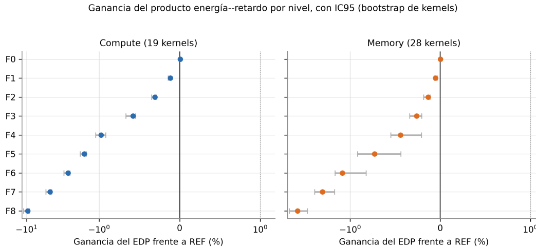
Figura 3.16: Misma información de la Tabla 3.16, en forma gráfica. El eje horizontal es simétrico-logarítmico para mostrar a la vez F0, cercano a cero, y F8, con una pérdida de casi un orden de magnitud. Ningún nivel deja el intervalo de confianza por encima de cero de forma útil. Fuente: elaboración propia.
