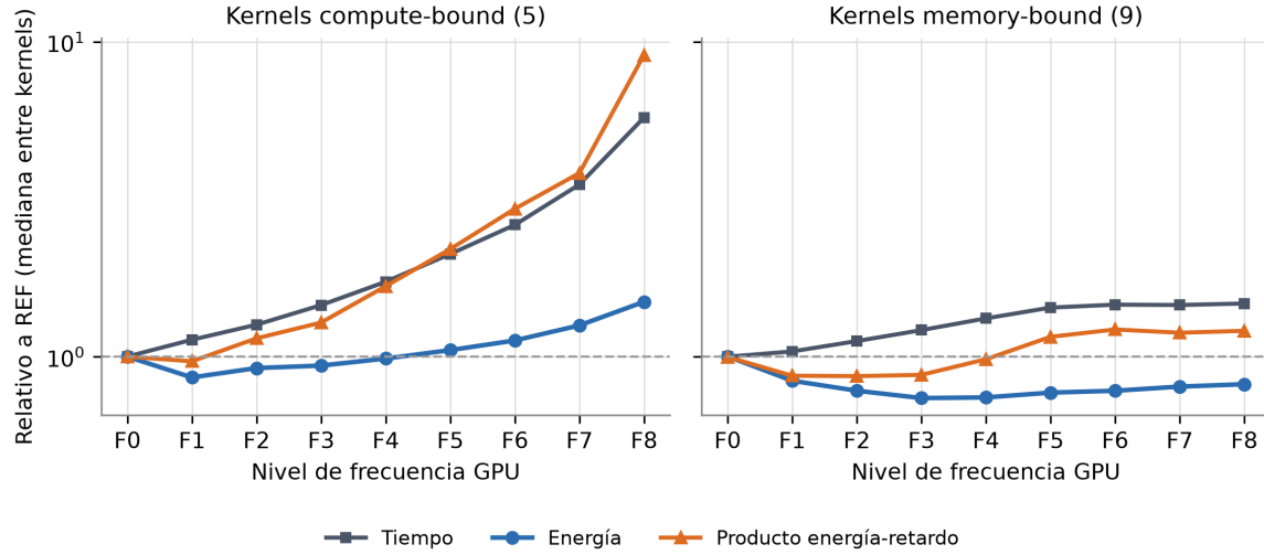
Figura 3.26: Mediana entre kernels del tiempo, la energía y el producto energía-retardo de cada nivel, relativos a REF, para las dos clases (5 y 9 kernels con corridas en REF, kernel como unidad, descriptivo; la significancia se evalúa por familia en la Tabla 3.20). El eje vertical es logarítmico. Fuente: elaboración propia.
