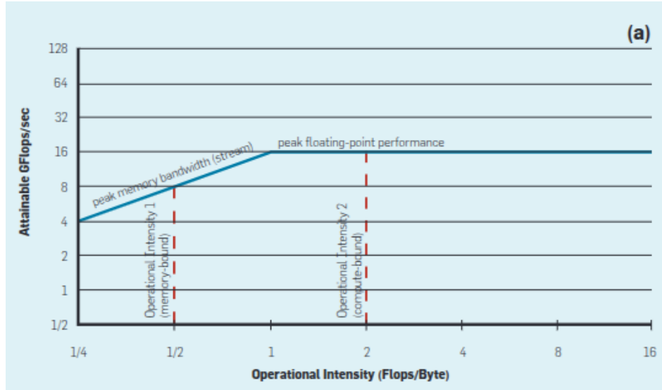
Figura 1.1: Modelo Roofline conceptual: relación entre el techo de ancho de banda de memoria y el techo de rendimiento de cómputo. Fuente: tomada de Williams et al. [42, Fig. 1(a)].
