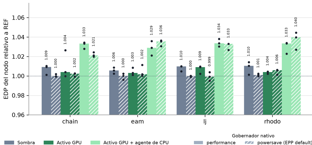
Figura 3.21: EDP del nodo de LAMMPS por entrada y brazo, relativo a la REF de su gobernador, bajo performance (barras lisas) y powersave (barras rayadas); la barra es la mediana y los puntos, cada bloque. Fuente: elaboración propia.
