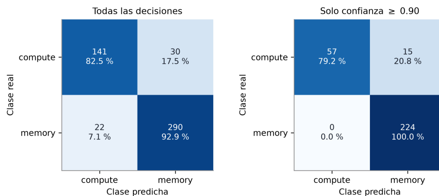
Figura 3.13: Matrices de confusión del modelo desplegado bajo validación por familia (483 corridas, una semilla; las métricas del texto por celda son promedios de cinco semillas). A la izquierda, todas las decisiones; a la derecha, solo las de confianza mayor o igual a 0.90. Fuente: elaboración propia.
