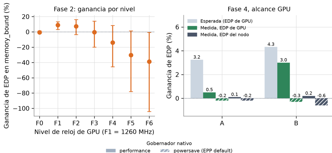
Figura 3.18: Izquierda: ganancia de EDP por nivel de reloj de GPU en fases memory_bound (Fase 2, IC95 sobre familias). Derecha: ganancia esperada de EDP de GPU (fracción de tiempo en memoria por la ganancia de F1) frente a la medida con el agente activo en el alcance GPU, en EDP de GPU y en EDP del nodo (medianas de tres repeticiones), bajo performance (barras lisas) y powersave (barras rayadas). Fuente: elaboración propia.
