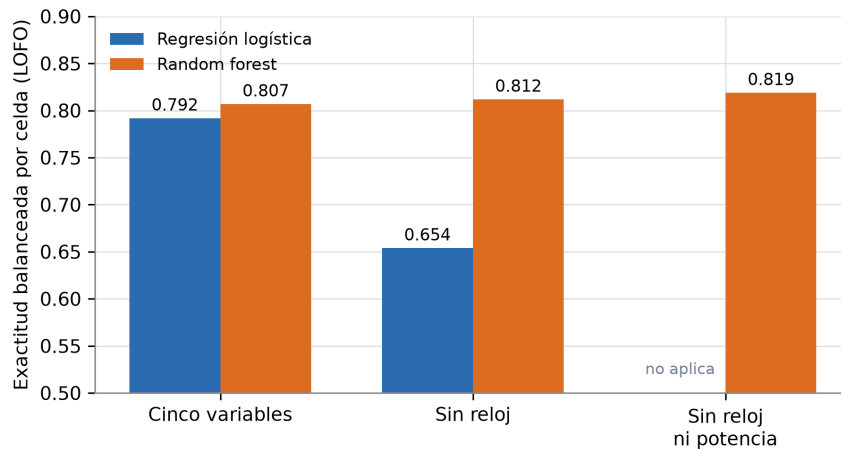
Figura 3.12: Exactitud balanceada por celda (LOFO, 483 corridas, 16 familias) al excluir las variables que dependen de la acción del agente. Fuente: elaboración propia.
