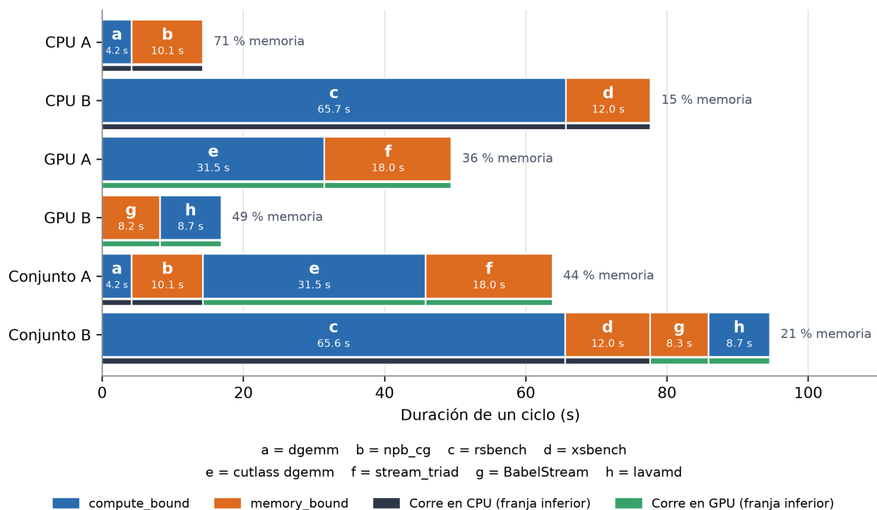
Figura 3.16: Un ciclo de cada aplicación, por fase (letra del kernel, clave debajo; color según su clase; franja inferior según el dispositivo). A la derecha, la fracción del ciclo en fases memory_bound . Fuente: elaboración propia.
