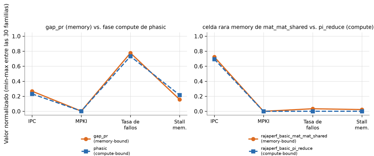
Figura 3.7: Cuatro variables de entrada, normalizadas al rango de las 30 familias, para los dos pares de celdas más confusables entre clases opuestas. Fuente: elaboración propia.
