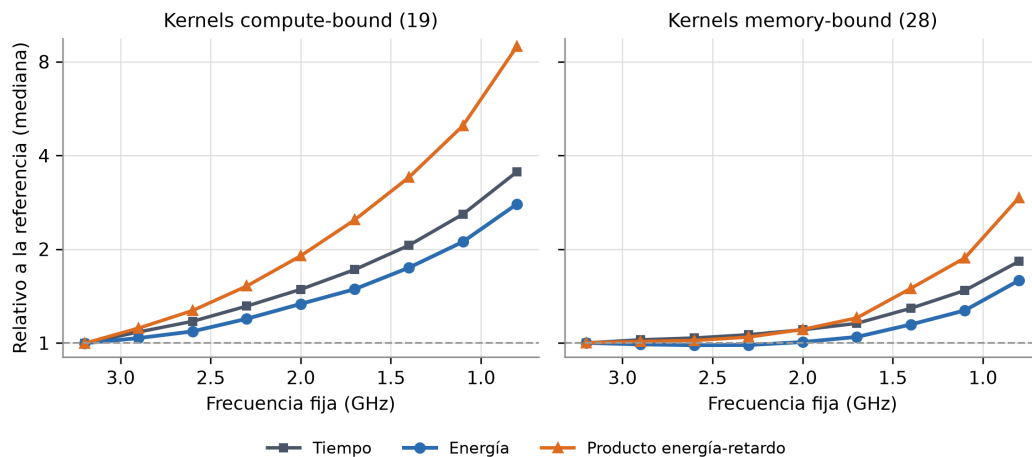
Figura 3.9: Mediana entre kernels de la energía (paquete y DRAM), el tiempo y el EDP de cada nivel fijo de CPU, relativos a la referencia nativa, para las dos clases. El eje vertical es logarítmico. Fuente: elaboración propia.
