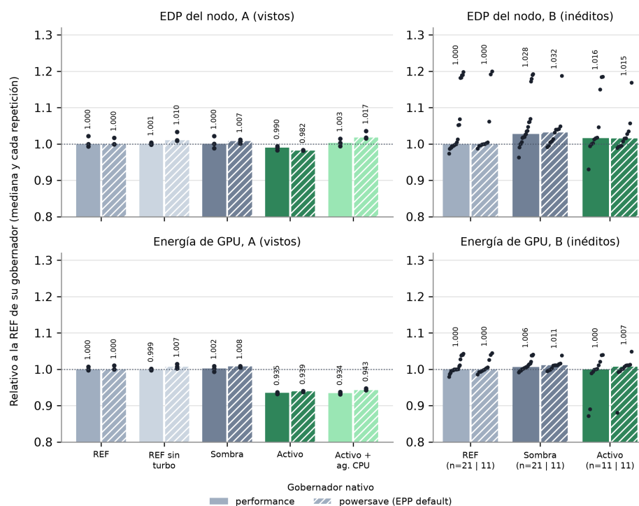
Figura 3.19: Escenario E. EDP del nodo (arriba) y energía de GPU (abajo), con la mediana (barra) y cada repetición (punto), para familias vistas (A) e inéditas (B), bajo performance (barras lisas) y powersave con EPP default (barras rayadas), cada uno frente a la REF de su gobernador. En B se agrupan las repeticiones de las corridas con la misma configuración; bajo cada brazo, el número de repeticiones de cada gobernador. Fuente: elaboración propia.
