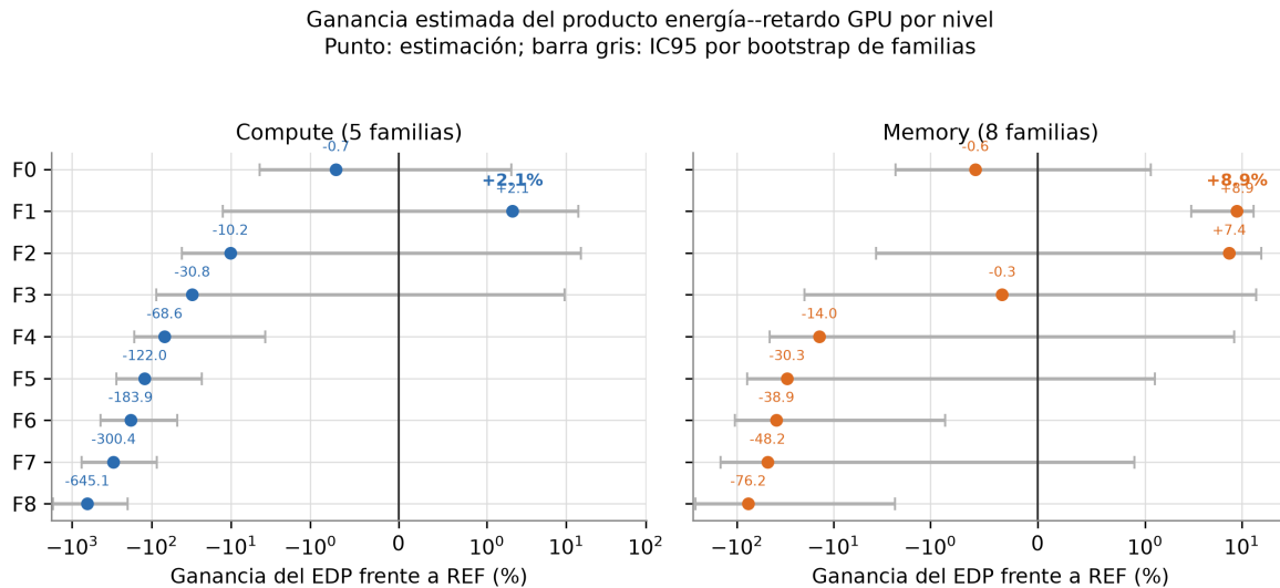
Figura 3.14: Ganancia del EDP GPU frente a la base por nivel y clase, con la familia como unidad (cómputo: 5 familias; memoria: 8). Cada punto es la ganancia estimada (en %, con su valor rotulado) y la barra gris, su IC95 por bootstrap , cuyos límites numéricos están en el repositorio; el rótulo en negrita señala F1. Valor p de la prueba pareada: en cómputo entre 0.438 y 1.000; en memoria, 0.020 en F1, 0.156 en F2 y entre 0.422 y 0.926 en los demás niveles. El eje horizontal es simétrico-logarítmico para mostrar a la vez F1, cercano a cero, y F8, con pérdidas de más de un orden de magnitud en compute_bound . Fuente: elaboración propia.
