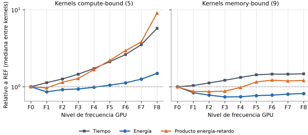
Figura 3.15: Mediana entre kernels del tiempo, la energía y el EDP de cada nivel de reloj de GPU, relativos a la base, para las dos clases (5 y 9 kernels con corridas en la base, kernel como unidad, descriptivo). El eje vertical es logarítmico. Fuente: elaboración propia.
