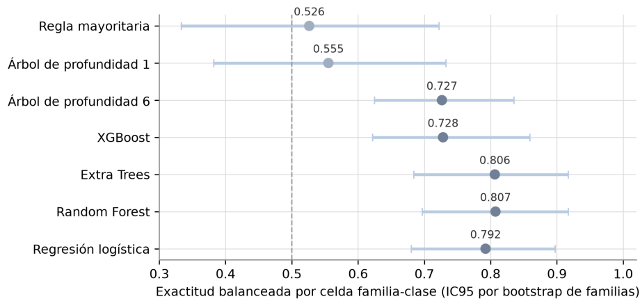
Figura 3.11: Exactitud balanceada por celda familia-clase de los siete modelos candidatos con las cinco señales, con intervalo de confianza del 95 % por bootstrap de familias. Fuente: elaboración propia.
