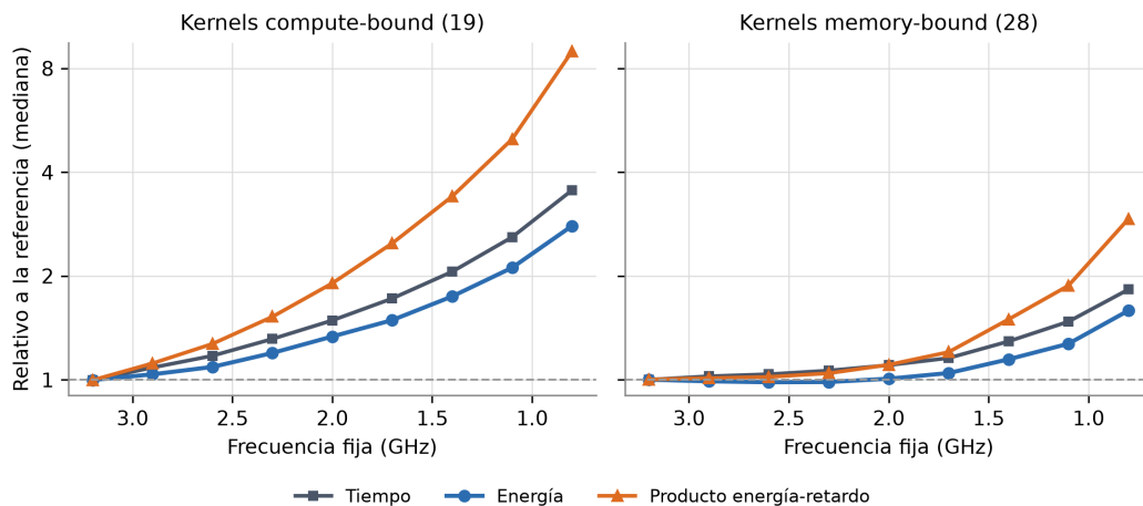
Figura A.1: Mediana entre kernels de la energía (paquete y DRAM), el tiempo y el EDP de cada nivel fijo de CPU, relativos a la referencia nativa, para las dos clases. El eje vertical es logarítmico. Fuente: elaboración propia.
