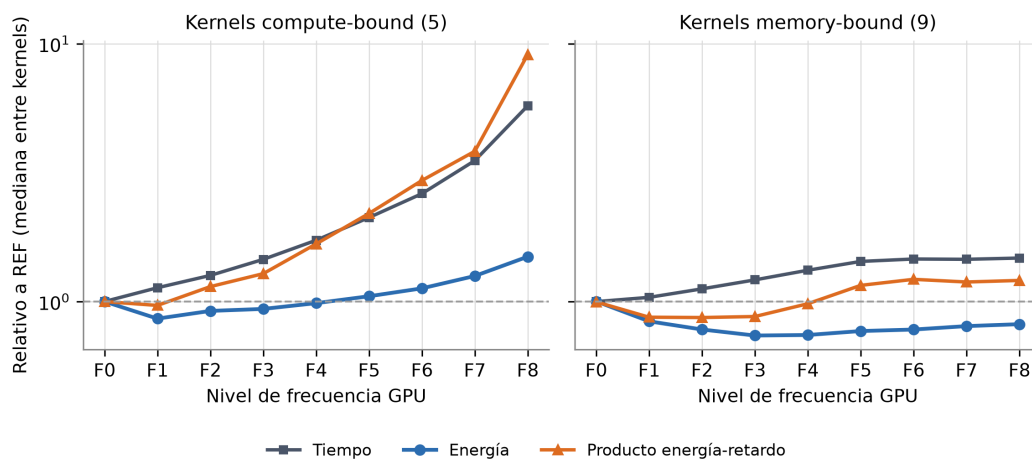
Figura A.2: Mediana entre kernels del tiempo, la energía y el EDP de cada nivel de reloj de GPU, relativos a la base, para las dos clases (5 y 9 kernels con corridas en la base, kernel como unidad, descriptivo). El eje vertical es logarítmico. Fuente: elaboración propia.
