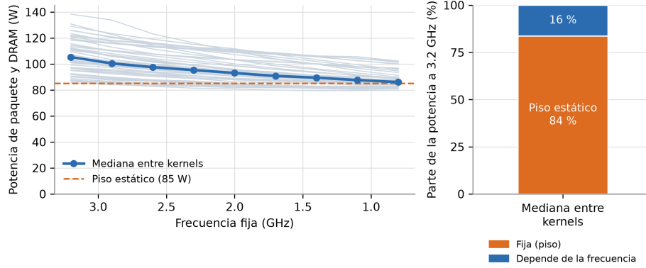
Figura 3.9: A la izquierda, potencia media de paquete y DRAM de cada kernel (líneas grises) y su mediana en cada nivel fijo, con el piso estático ajustado. A la derecha, parte de la potencia a 3.2 GHz que corresponde al piso: la barra muestra la mediana entre kernels (84 %), y según el kernel va de 62 a 94 %. Fuente: elaboración propia.
