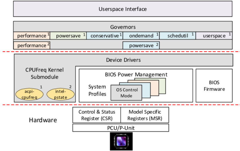
Figura 1.3: Jerarquía mediante la cual una política de rendimiento solicita cambios que posteriormente son materializados por el hardware. Fuente: Tomado de Hebbar y Milenković [22].
