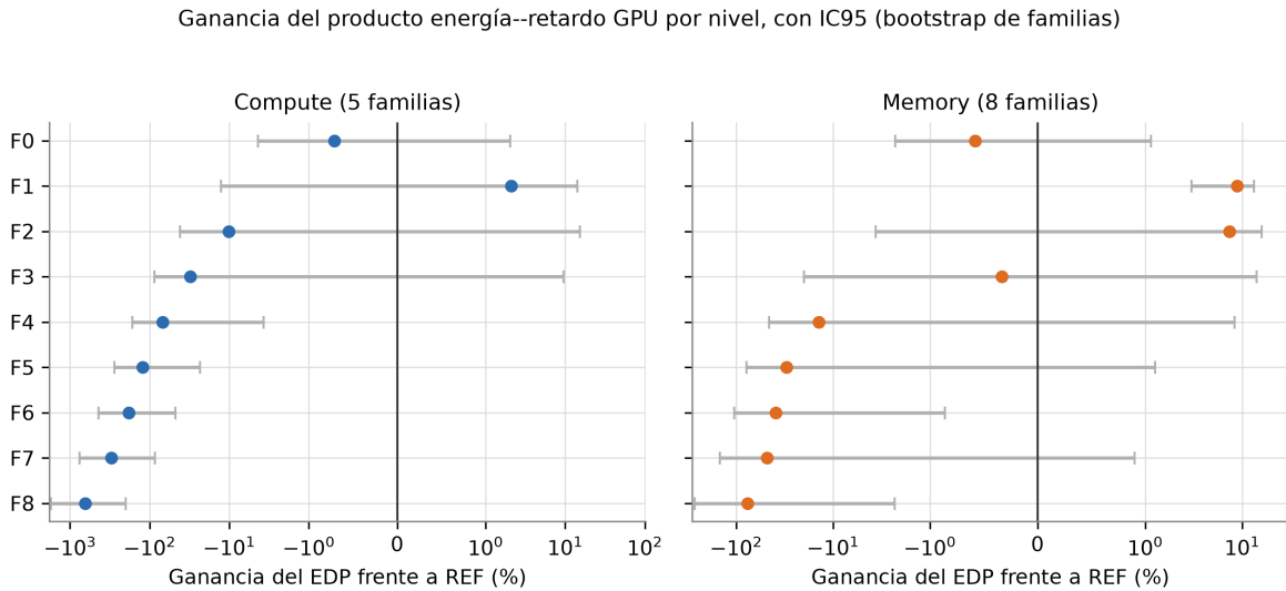
Figura 3.25: Misma información de la Tabla 3.19, en forma gráfica, con la familia como unidad. El eje horizontal es simétrico-logarítmico para mostrar a la vez F1, cercano a cero, y F8, con pérdidas de más de un orden de magnitud en compute_bound . Fuente: elaboración propia.
