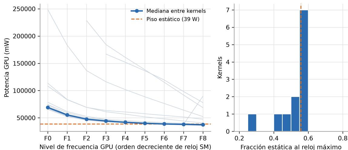
Figura 3.27: Izquierda: potencia media de GPU de cada kernel (líneas grises) y su mediana en cada nivel, con el piso estático ajustado (12 kernels con ajuste identificable). Derecha: distribución entre esos kernels de la fracción de la potencia al reloj más alto que corresponde al piso. Fuente: elaboración propia.
