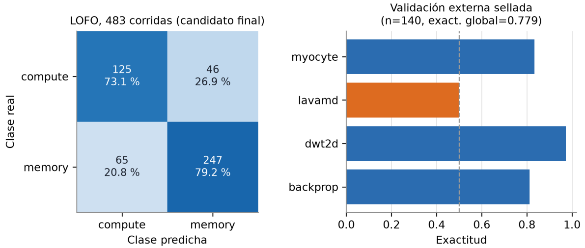
Figura 3.24: Izquierda: matriz de confusión agregada del candidato final bajo leave-one-familia-out (483 corridas). Derecha: exactitud por familia en la validación externa sellada (Backprop, DWT2D, LavaMD, Myocyte; 140 corridas nunca usadas en ninguna decisión de esta ronda). Fuente: elaboración propia.
