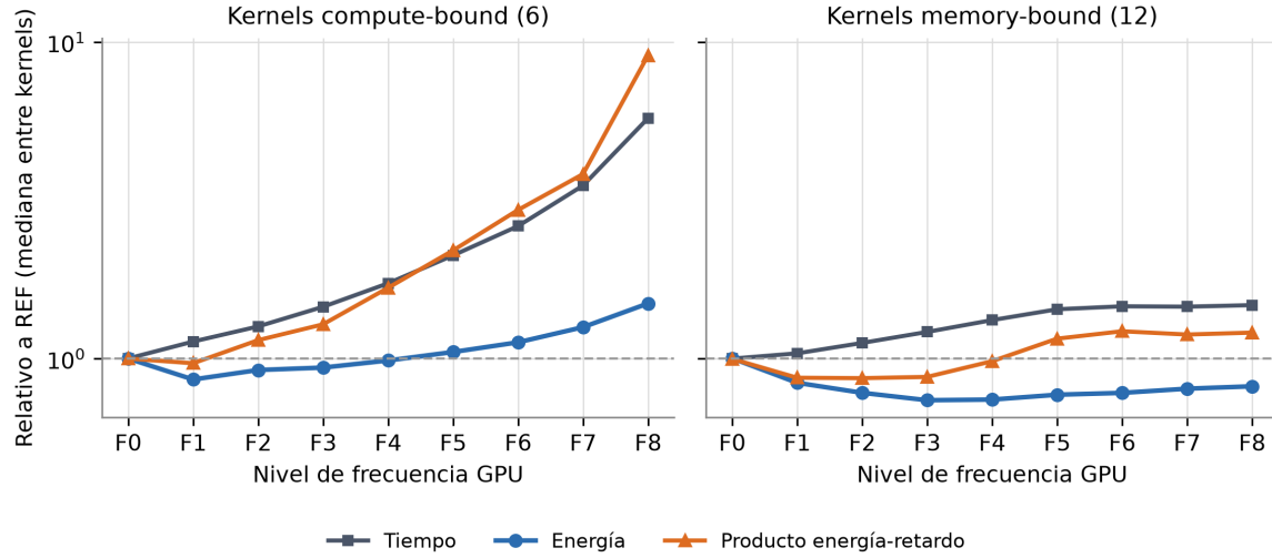
Figura 3.26: Mediana entre kernels del tiempo, la energía y el producto energía-retardo de cada nivel, relativos a REF, para las dos clases (18 kernels, kernel como unidad, descriptivo; la significancia se evalúa por familia en la Tabla 3.19). El eje vertical es logarítmico. Fuente: elaboración propia.
