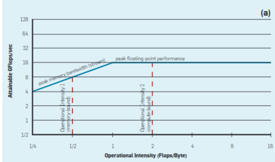
Figura 1.1: Modelo Roofline conceptual: relación entre el techo de ancho de banda de memoria y el techo de rendimiento de cómputo. Fuente: tomado de Williams et al. [68, Fig. 1(a)].
