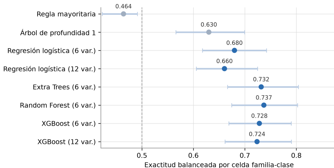
Figura 3.5: Exactitud balanceada por celda de familia y clase de cada modelo, con intervalo de confianza del 95 % obtenido por remuestreo de las 30 familias. Los intervalos se solapan entre todos los modelos con capacidad suficiente. Nota. Elaboración propia.
