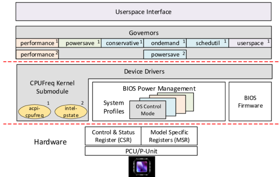
Figura 1.8: Jerarquía de los mecanismos de gestión de rendimiento desde la interfaz de espacio de usuario hasta el hardware. Fuente: tomado de Hebbar y Milenković [29].
