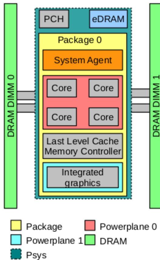
Figura 1.6: Dominios energéticos expuestos mediante Intel RAPL. Fuente: tomado de Thamm y Leser [62].
