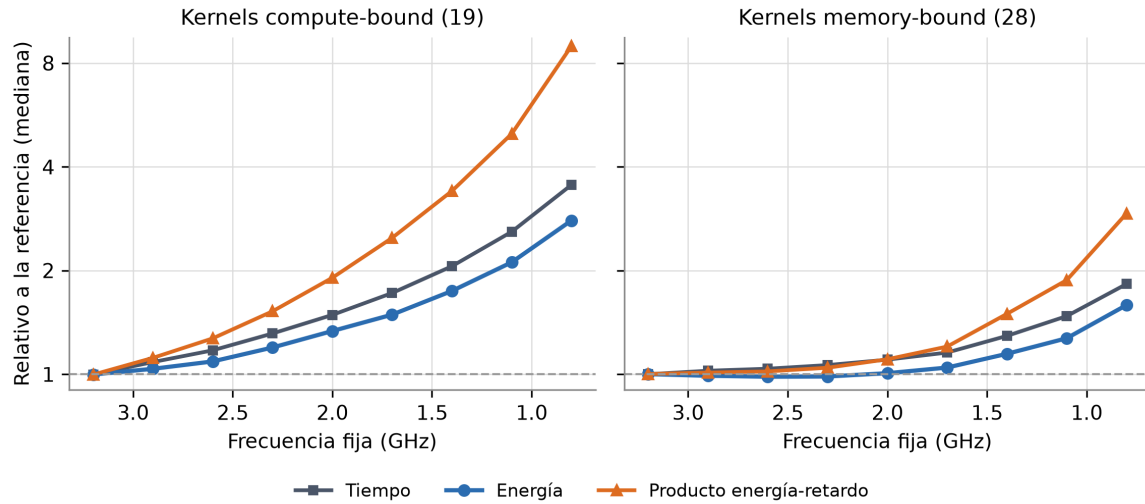
Figura 3.12: Mediana entre kernels de la energía (paquete y DRAM), el tiempo y el producto energía-retardo de cada nivel fijo, relativos a la referencia nativa, para las dos clases. El eje vertical es logarítmico. Nota. Elaboración propia.
