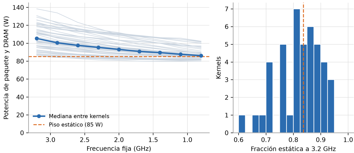
Figura 3.13: A la izquierda, potencia media de paquete y DRAM de cada kernel (líneas grises) y su mediana en cada nivel fijo, con el piso estático ajustado. A la derecha, distribución entre kernels de la fracción de la potencia a 3.2 GHz que corresponde al piso. Nota. Elaboración propia.
