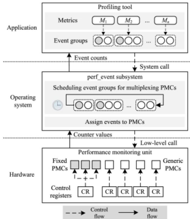
Figura 1.5: Flujo de configuración y lectura de eventos de rendimiento mediante el subsistema perf_event de Linux. Fuente: tomado de Liu et al. [50].
