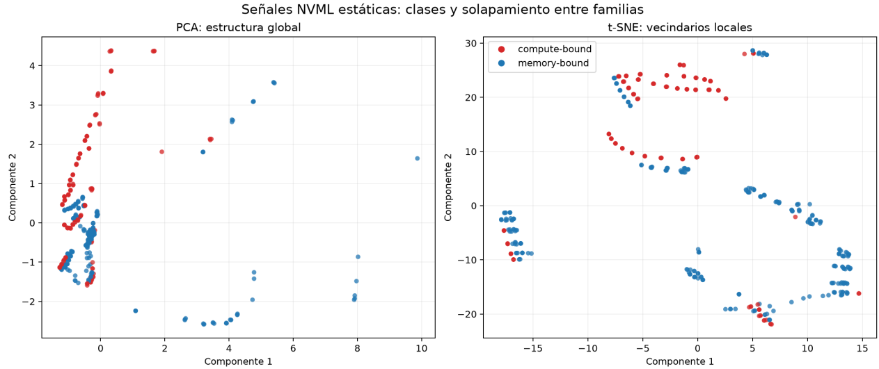
Figura 3.15: Proyecciones PCA y t-SNE de las medianas e IQR de utilización GPU, utilización de memoria, potencia y reloj SM. La proyección t-SNE es diagnóstica y no se utiliza para medir generalización. Nota. Elaboración propia.
