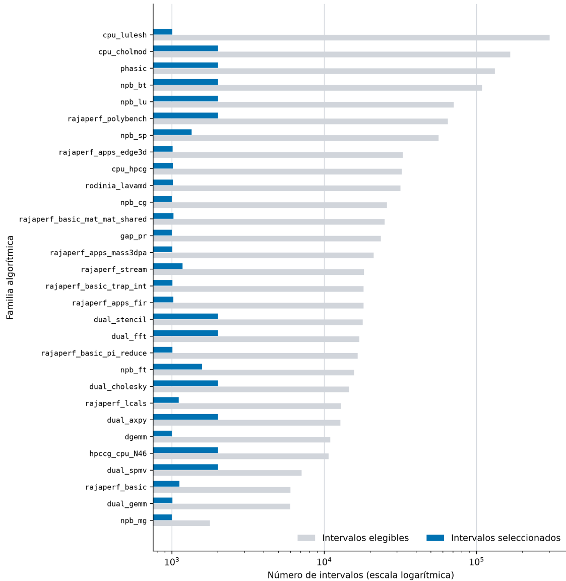
Figura 3.4: Intervalos elegibles y seleccionados por familia algorítmica. El eje logarítmico permite comparar familias cuyo volumen original difiere en varios órdenes de magnitud. Fuente: Elaboración propia.
