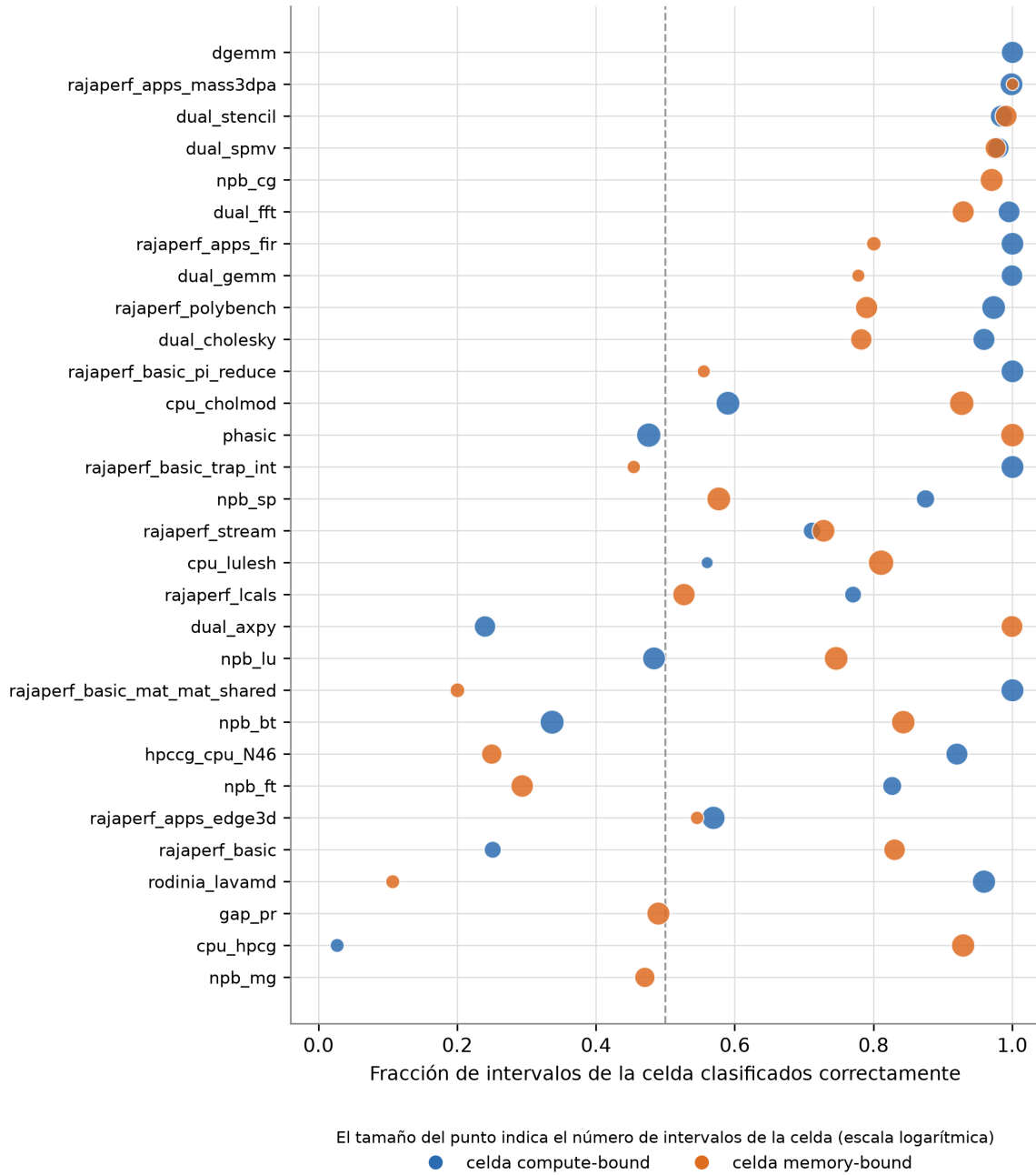
Figura 3.6: Fracción de aciertos del modelo final en cada una de las 56 celdas de familia y clase, con evaluación sobre todos los intervalos de la familia retirada. Las familias con una sola celda son las de una sola clase. Nota. Elaboración propia.
