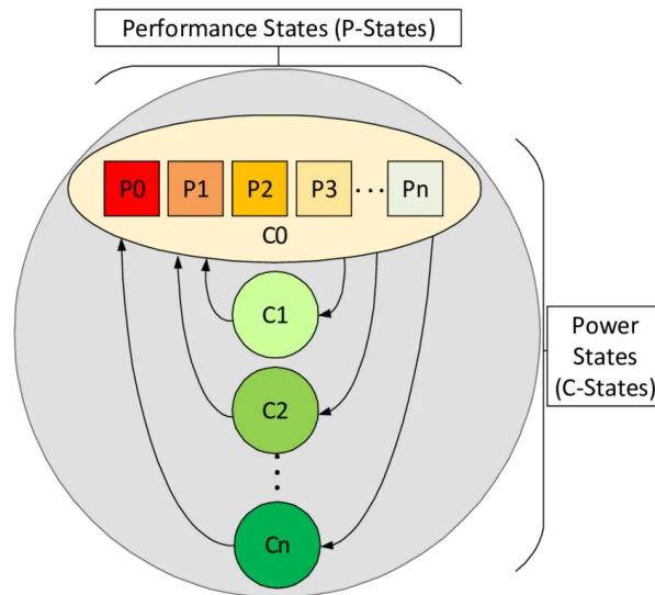
Figura 1.7: Relación conceptual entre estados de rendimiento (P-states) y estados de inactividad (C-states) del procesador. Fuente: tomado de Hebbar y Milenković [29].
