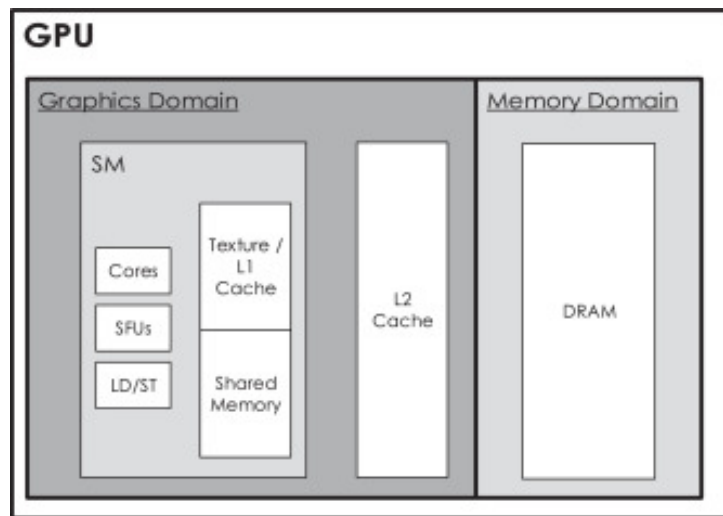
Figura 1.10: Representación conceptual de los dominios de procesamiento y memoria en una GPU. Fuente: tomado de Guerreiro et al. [28].
