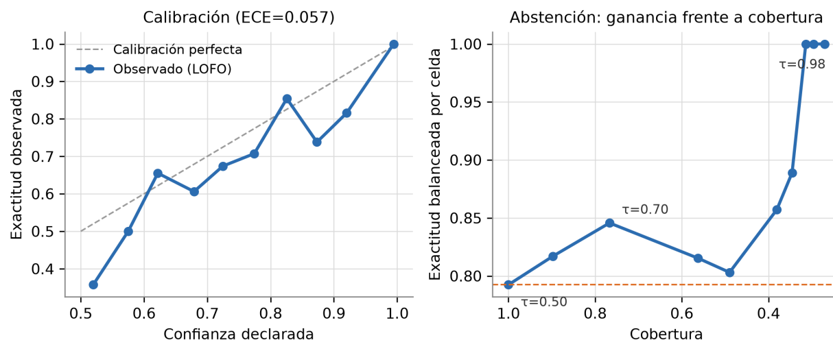
Figura 3.23: Izquierda: confianza declarada contra exactitud observada, diez cubetas de igual ancho. Derecha: exactitud balanceada por celda contra cobertura, para distintos umbrales de decisión \tau . Fuente: elaboración propia.
