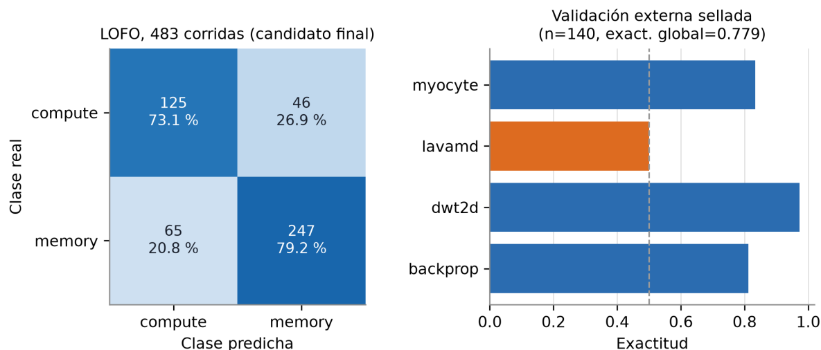
Figura 3.24: Izquierda: matriz de confusión agregada del candidato por desempeño bajo leave-one-family-out (483 corridas). Derecha: exactitud por familia en la validación externa sellada (Backprop, DWT2D, LavaMD, Myocyte; 140 corridas nunca usadas en ninguna decisión de esta ronda). Fuente: elaboración propia.
