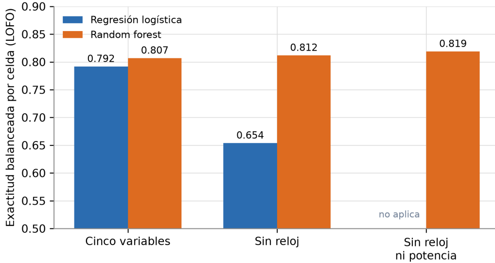
Figura 3.25: Exactitud balanceada por celda (LOFO, 483 corridas, 16 familias) al excluir las variables que dependen de la acción del agente. Fuente: elaboración propia.
