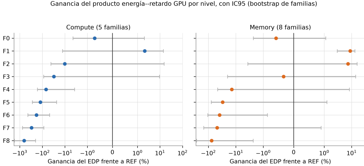
Figura 3.26: Misma información de la Tabla 3.20, en forma gráfica, con la familia como unidad. El eje horizontal es simétrico-logarítmico para mostrar a la vez F1, cercano a cero, y F8, con pérdidas de más de un orden de magnitud en compute_bound . Fuente: elaboración propia.
