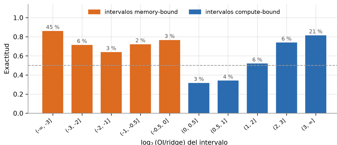
Figura 3.14: Exactitud del modelo final por franja de \log_2(\text{OI}/\text{ridge}) . El porcentaje sobre cada barra indica qué fracción de los intervalos cae en esa franja. Las franjas negativas corresponden a intervalos memory-bound y las positivas a compute-bound . Fuente: elaboración propia.
