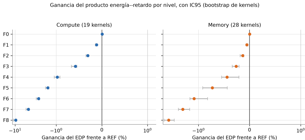
Figura 3.16: Misma información de la Tabla 3.16, en forma gráfica. El eje horizontal es simétrico-logarítmico para mostrar a la vez F0, cercano a cero, y F8, con una pérdida de casi un orden de magnitud. Ningún nivel deja el intervalo de confianza por encima de cero de forma útil. Fuente: elaboración propia.
