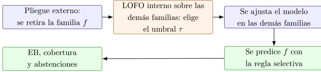
Figura 2.4: Validación anidada leave-one-family-out . La familia retirada no interviene en ninguna decisión de ajuste. Fuente: elaboración propia.
