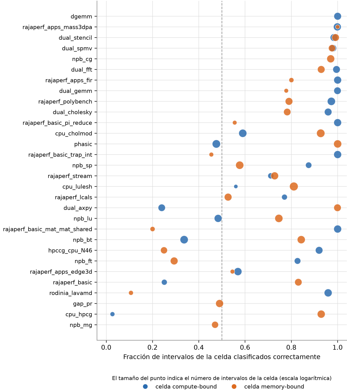
Figura 3.8: Fracción de aciertos del modelo final en cada una de las 56 celdas de familia y clase, con evaluación sobre todos los intervalos de la familia retirada. Las familias con una sola celda son las de una sola clase. Fuente: elaboración propia.
