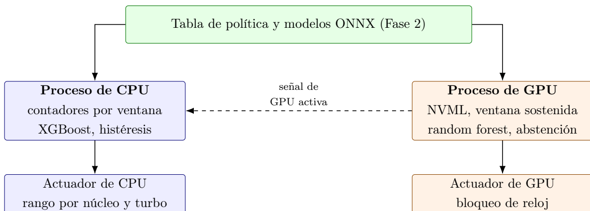
Figura 2.5: Arquitectura del agente: dos procesos, una tabla de política compartida y una señal de coordinación. Fuente: elaboración propia.
