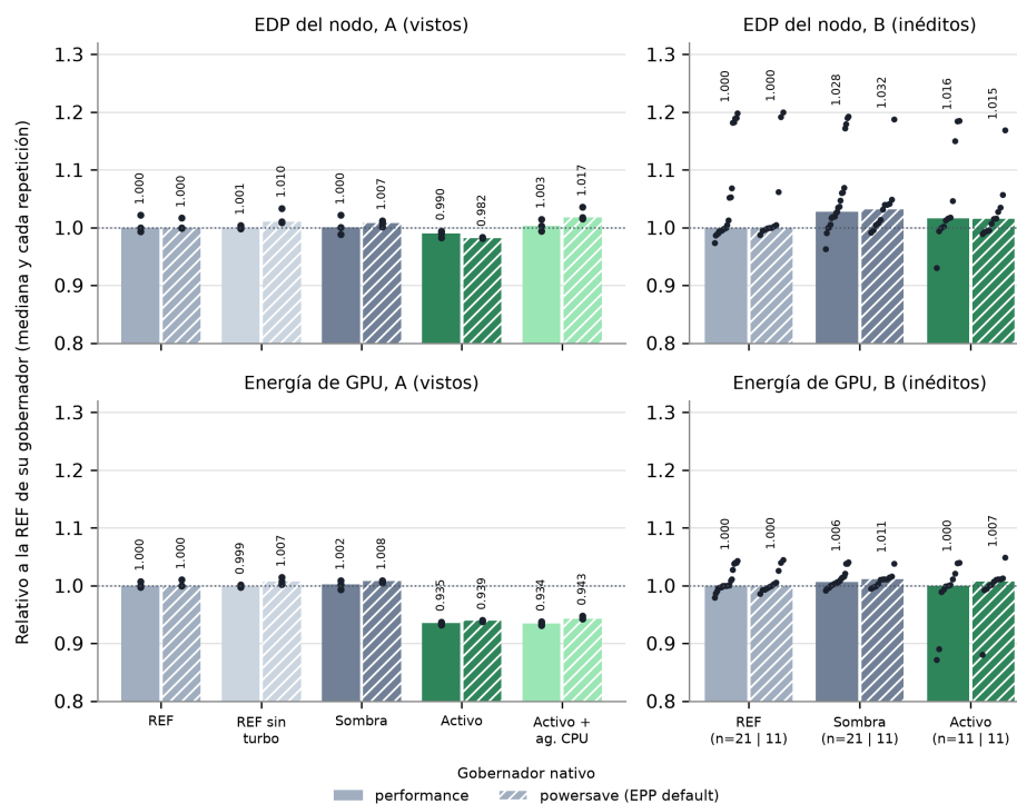
Figura 3.15: Escenario E. EDP del nodo (arriba) y energía de GPU (abajo), con la mediana (barra) y cada repetición (punto), para familias vistas (A) e inéditas (B), bajo performance (barras lisas) y powersave con EPP default (barras rayadas), cada uno frente a la REF de su gobernador. En B se agrupan las repeticiones de las corridas con la misma configuración; bajo cada brazo, el número de repeticiones de cada gobernador.
