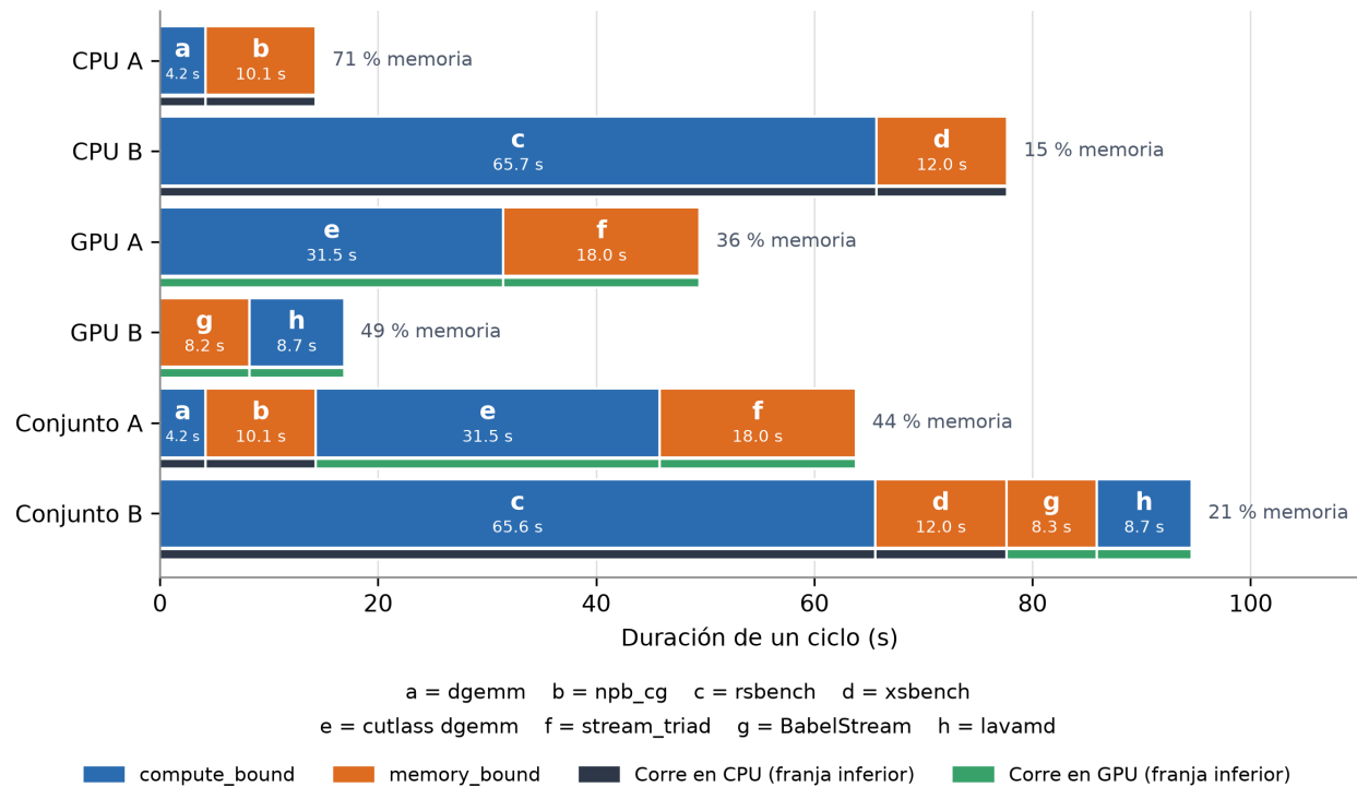
Figura 3.12: Un ciclo de cada aplicación, por fase (letra del kernel, clave debajo; color según su clase; franja inferior según el dispositivo). A la derecha, la fracción del ciclo en fases memory_bound . Fuente: elaboración propia.
