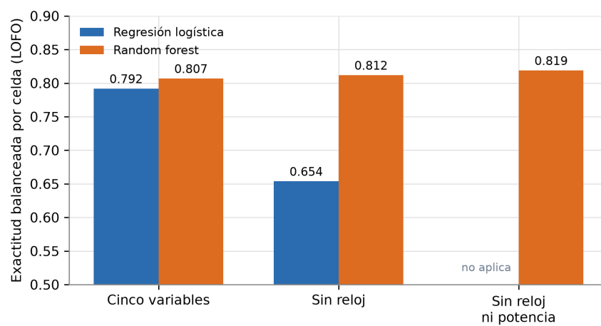
Figura A.4: Exactitud balanceada por celda (LOFO, 483 corridas, 16 familias) al excluir las variables que dependen de la acción del agente. Fuente: elaboración propia.
