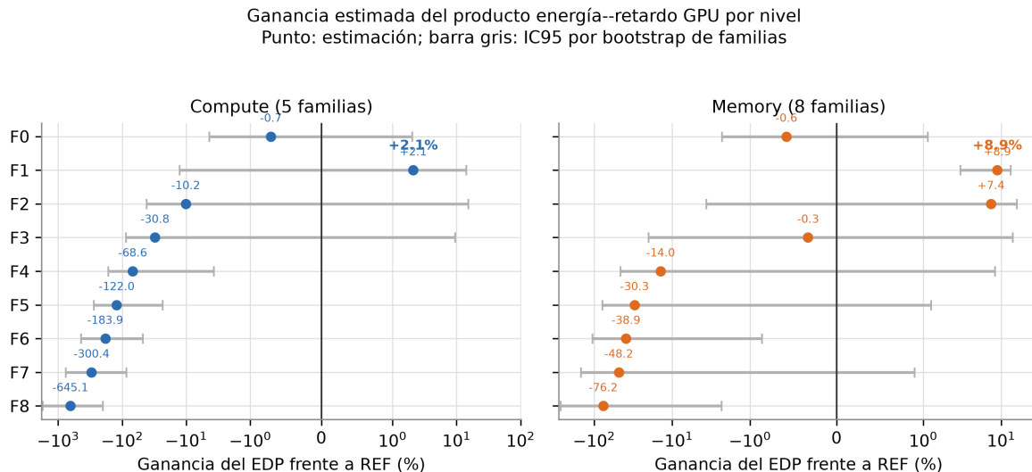
Figura 3.11: Ganancia del EDP GPU frente a la base por nivel y clase, con la familia como unidad (cómputo: 5 familias; memoria: 8). Cada punto es la ganancia estimada (en %, con su valor rotulado) y la barra gris, su IC95 por bootstrap , cuyos límites numéricos están en el repositorio; el rótulo en negrita señala F1. Valor p de la prueba pareada: en cómputo entre 0.438 y 1.000; en memoria, 0.020 en F1, 0.156 en F2 y entre 0.422 y 0.926 en los demás niveles. El eje horizontal es simétrico-logarítmico para mostrar a la vez F1, cercano a cero, y F8, con pérdidas de más de un orden de magnitud en compute_bound . Fuente: elaboración propia.
