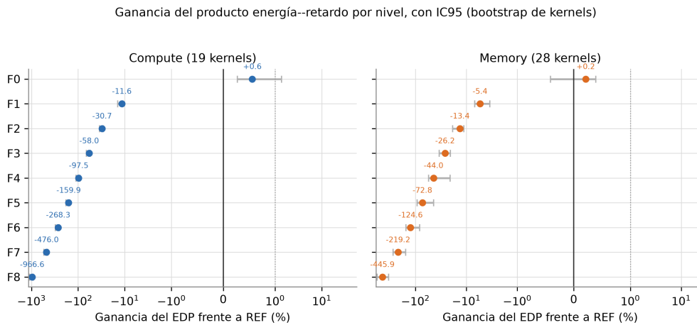
Figura 3.7: Ganancia del EDP frente a la base por nivel y clase (cómputo: 19 kernels; memoria: 28), con IC95 por bootstrap de kernels; eje simétrico-logarítmico. Valores p y límites numéricos en el material complementario. Fuente: elaboración propia.
