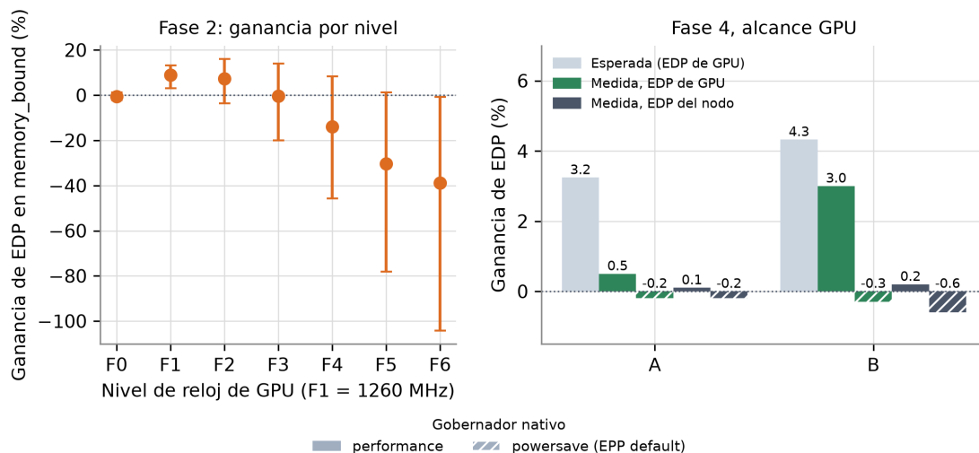
Figura 3.14: Izquierda: ganancia de EDP por nivel de reloj de GPU en fases memory_bound (Fase 2, IC95 sobre familias). Derecha: ganancia esperada de EDP de GPU (fracción de tiempo en memoria por la ganancia de F1) frente a la medida con el agente activo en el alcance GPU, en EDP de GPU y en EDP del nodo (medianas de tres repeticiones), bajo performance (barras lisas) y powersave (barras rayadas).
