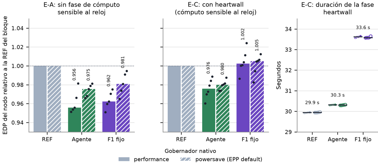
Figura 3.16: Agente frente a F1 fijo. EDP del nodo relativo a la REF del mismo bloque en E-A, bajo performance (barras lisas) y powersave (barras rayadas), y lo mismo en E-C; la barra es la mediana y los puntos, cada bloque. A la derecha, duración de la fase de heartwall en E-C por brazo, bajo performance (puntos llenos) y powersave (puntos vacíos), con la mediana como línea. Fuente: elaboración propia.
