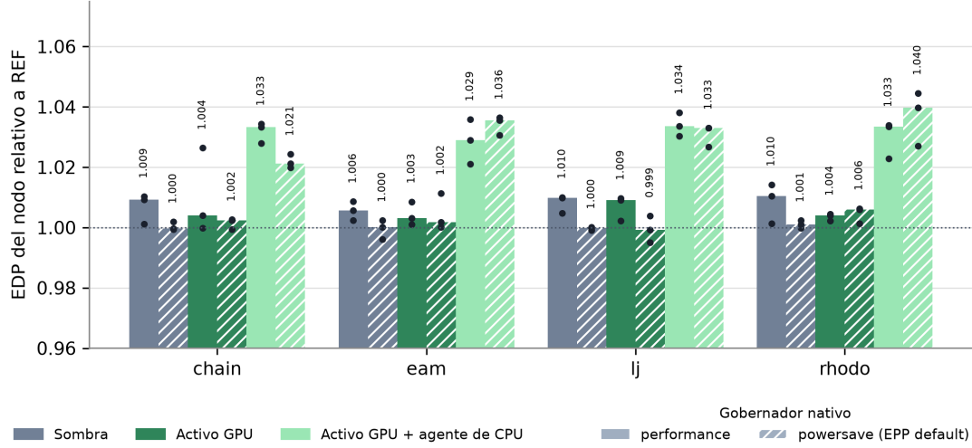
Figura 3.17: EDP del nodo de LAMMPS por entrada y brazo, relativo a la REF de su gobernador, bajo performance (barras lisas) y powersave (barras rayadas); la barra es la mediana y los puntos, cada bloque. Fuente: elaboración propia.
