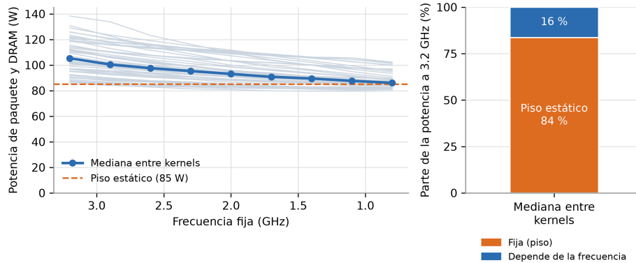
Figura 3.8: A la izquierda, potencia media de paquete y DRAM de cada kernel (líneas grises) y su mediana en cada nivel fijo, con el piso estático ajustado. A la derecha, parte de la potencia a 3.2 GHz que corresponde al piso: la barra muestra la mediana entre kernels (84 %), y según el kernel va de 62 a 94 %. Fuente: elaboración propia.
