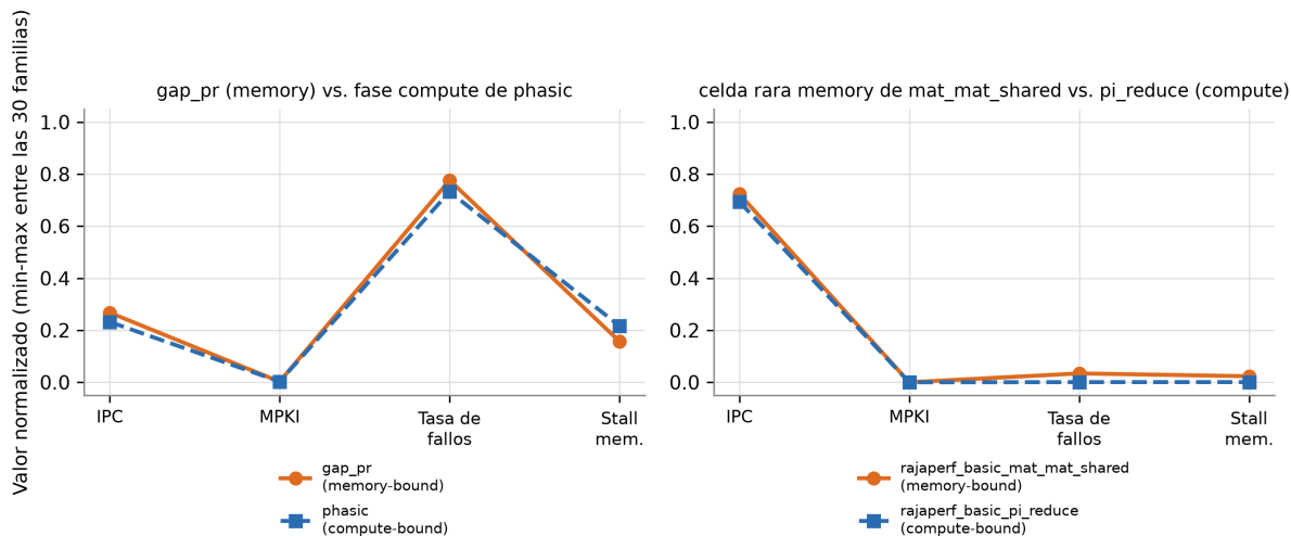
Figura A.3: Cuatro variables de entrada, normalizadas al rango de las 30 familias, para los dos pares de celdas más confusables entre clases opuestas. Fuente: elaboración propia.
