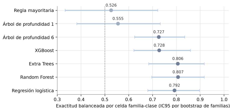
Figura 3.9: Exactitud balanceada por celda familia-clase de los siete modelos candidatos con las cinco señales, con intervalo de confianza del 95 % por bootstrap de familias. Fuente: elaboración propia.
