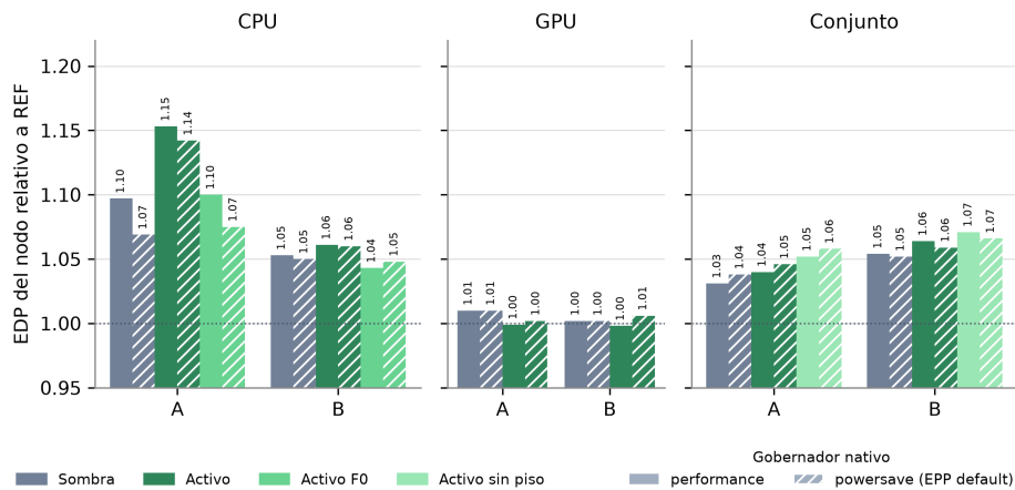
Figura 3.13: EDP del nodo, (E_{\text{CPU}} + E_{\text{GPU}})T , relativo a la REF de su gobernador, por alcance, aplicación (A: vistos, B: inéditos) y brazo, en la matriz inicial, bajo performance (barras lisas) y powersave con EPP default (barras rayadas). La línea punteada marca la paridad con la REF.
