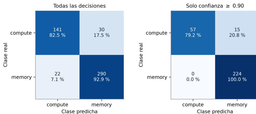
Figura 3.10: Matrices de confusión del modelo desplegado bajo validación por familia (483 corridas, una semilla; las métricas del texto por celda son promedios de cinco semillas). A la izquierda, todas las decisiones; a la derecha, solo las de confianza mayor o igual a 0.90. Fuente: elaboración propia.
