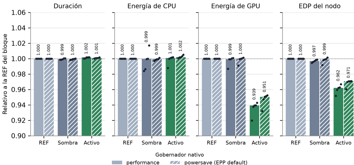
Figura 3.18: CloverLeaf CUDA Fortran: duración, energía de CPU, energía de GPU y EDP del nodo de cada brazo relativos a la REF de su bloque, bajo performance (barras lisas) y powersave (barras rayadas). La barra es la mediana de los cinco bloques, los puntos son los bloques individuales y la línea punteada marca la paridad con la base. Fuente: elaboración propia.
