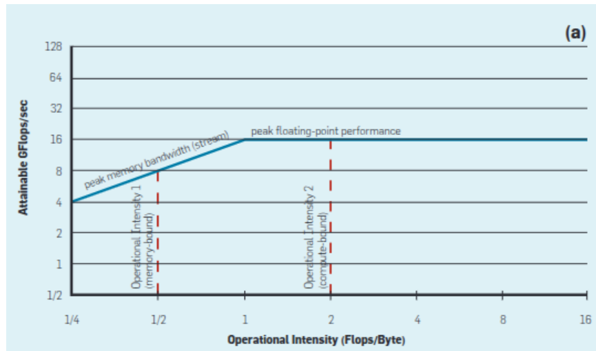
Figura 1.1: Modelo Roofline conceptual con el techo de ancho de banda de memoria y el techo de rendimiento de cómputo. Nota. Tomado de Williams et al. [40, Fig. 1(a)].
