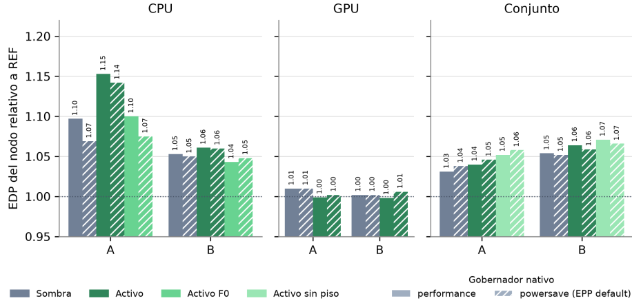
Figura 3.17: EDP del nodo, (E_{CPU} + E_{GPU})T , relativo a la REF de su gobernador, por alcance, aplicación (A: vistos, B: inéditos) y brazo, en la matriz inicial, bajo performance (barras lisas) y powersave con EPP default (barras rayadas). La línea punteada marca la paridad con la REF. Fuente: elaboración propia.
