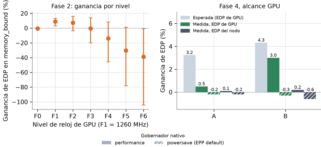
Figura 3.18: Izquierda: ganancia de EDP por nivel de reloj de GPU en fases memory_bound (Fase 2, IC95 sobre familias). Derecha: ganancia esperada de EDP de GPU (fracción de tiempo en memoria por la ganancia de F1) frente a la medida con el agente activo en el alcance GPU, en EDP de GPU y en EDP del nodo (medianas de tres repeticiones), bajo performance (barras lisas) y powersave (barras rayadas). Fuente: elaboración propia.
