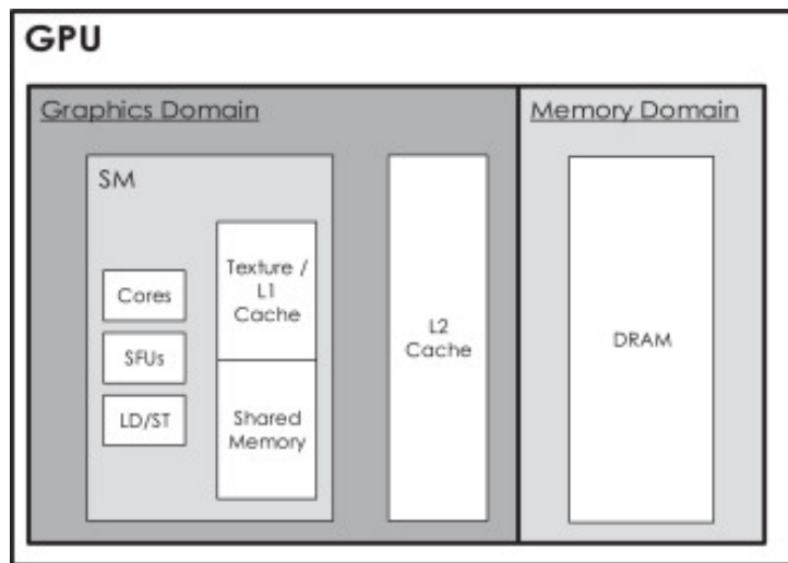
Figura 1.10: Representación conceptual de los dominios de procesamiento y memoria en una GPU. Fuente: tomado de Guerreiro et al. [21].
