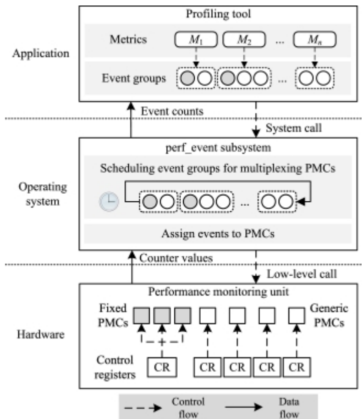
Figura 1.5: Flujo de configuración y lectura de eventos de rendimiento mediante el subsistema perf_event de Linux. Fuente: tomado de Liu et al. [39].
