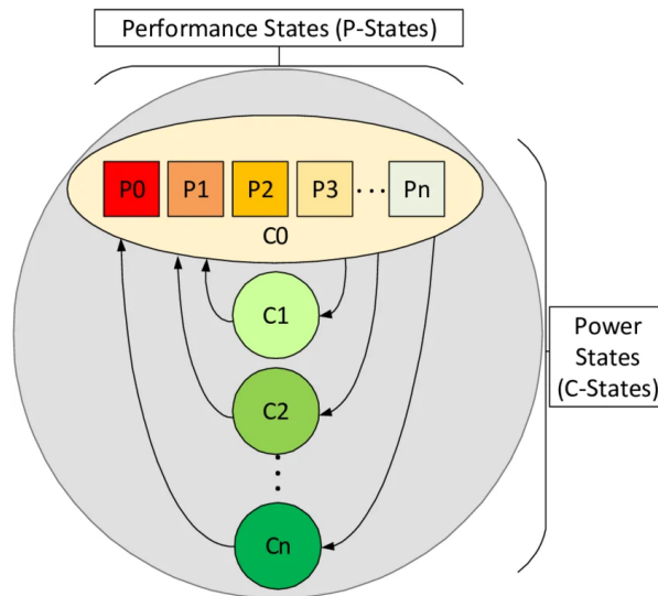
Figura 1.7: Relación conceptual entre estados de rendimiento (P-states) y estados de inactividad (C-states) del procesador. Fuente: tomado de Hebbar y Milenković [22].
