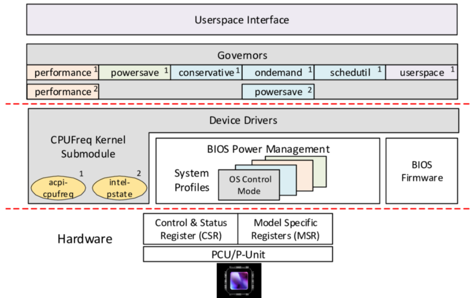
Figura 1.8: Jerarquía de los mecanismos de gestión de rendimiento desde la interfaz de espacio de usuario hasta el hardware. Fuente: tomado de Hebbar y Milenković [22].
