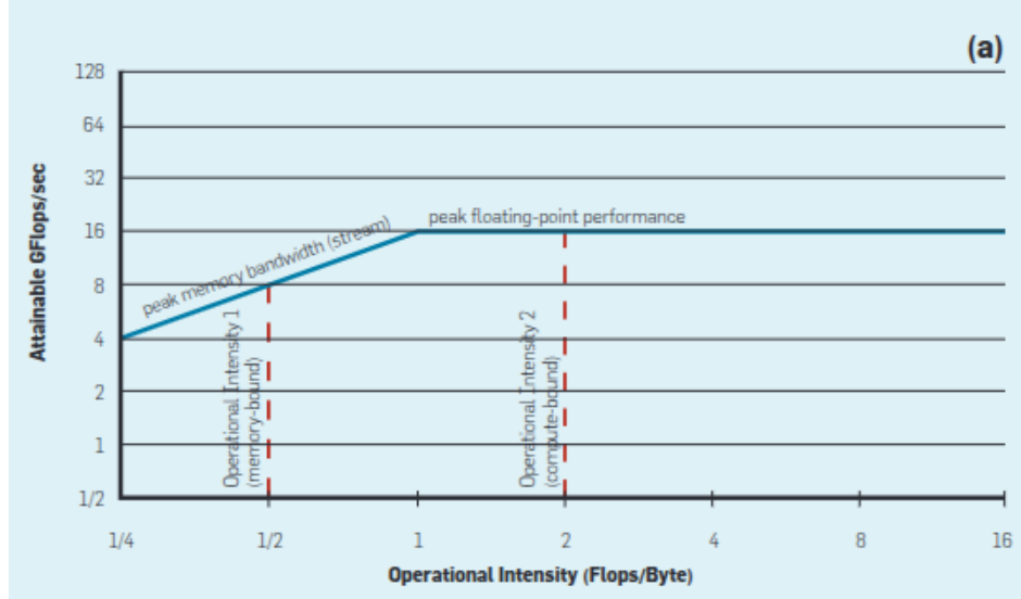
Figura 1.1: Modelo Roofline conceptual: relación entre el techo de ancho de banda de memoria y el techo de rendimiento de cómputo. Fuente: tomado de Williams et al. [56, Fig. 1(a)].
