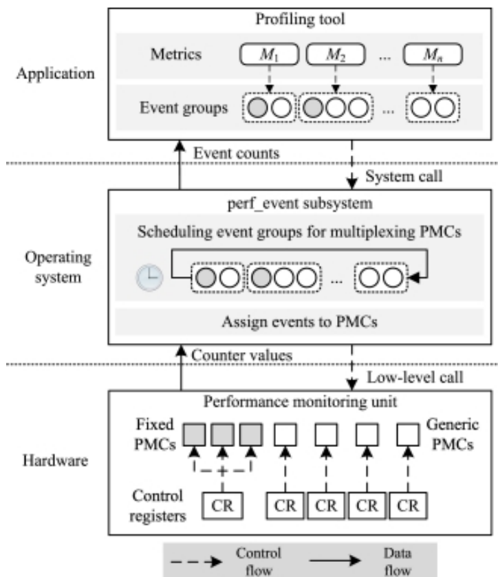
Figura 1.5: Flujo de configuración y lectura de eventos de rendimiento mediante el subsistema perf_event de Linux. Fuente: tomado de Liu et al. [40].
