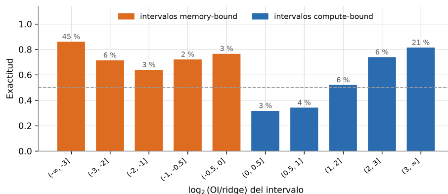
Figura 3.12: Exactitud del modelo final por franja de \log_2(\text{OI/ridge}) . El porcentaje sobre cada barra indica qué fracción de los intervalos cae en esa franja. Las franjas negativas corresponden a intervalos memory-bound y las positivas a compute-bound . Fuente: elaboración propia.
