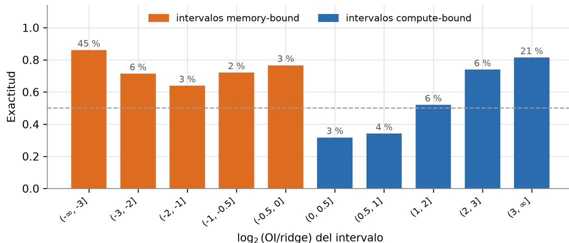
Figura 3.10: Exactitud del modelo final por franja de \log_2(\text{OI/ridge}) . El porcentaje sobre cada barra indica qué fracción de los intervalos cae en esa franja. Las franjas negativas corresponden a intervalos memory-bound y las positivas a compute-bound . Nota. Elaboración propia.
