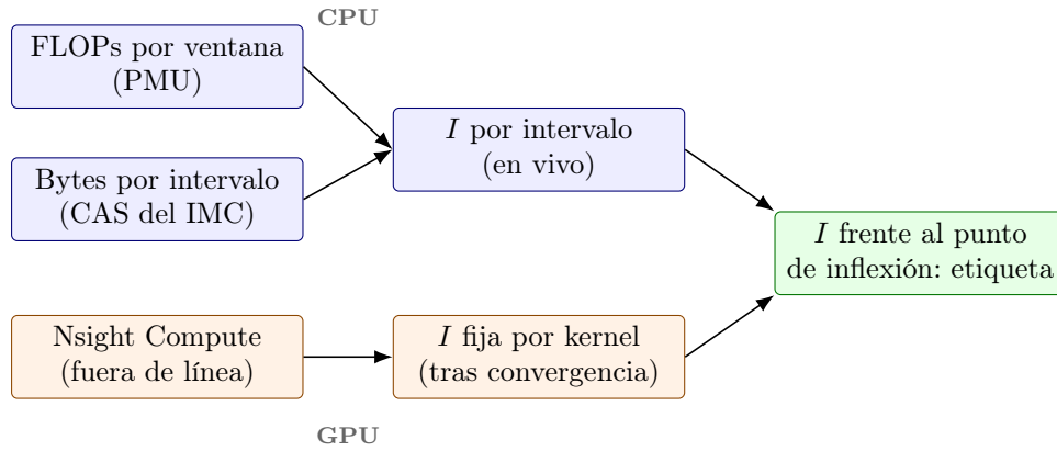
Figura 2.3: Obtención de la intensidad operacional y de la etiqueta Roofline en CPU y GPU.
