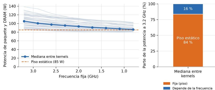
Figura 3.10: A la izquierda, potencia media de paquete y DRAM de cada kernel (líneas grises) y su mediana en cada nivel fijo, con el piso estático ajustado. A la derecha, parte de la potencia a 3.2 GHz que corresponde al piso: la barra muestra la mediana entre kernels (84 %), y según el kernel va de 62 a 94 %. Fuente: elaboración propia.
