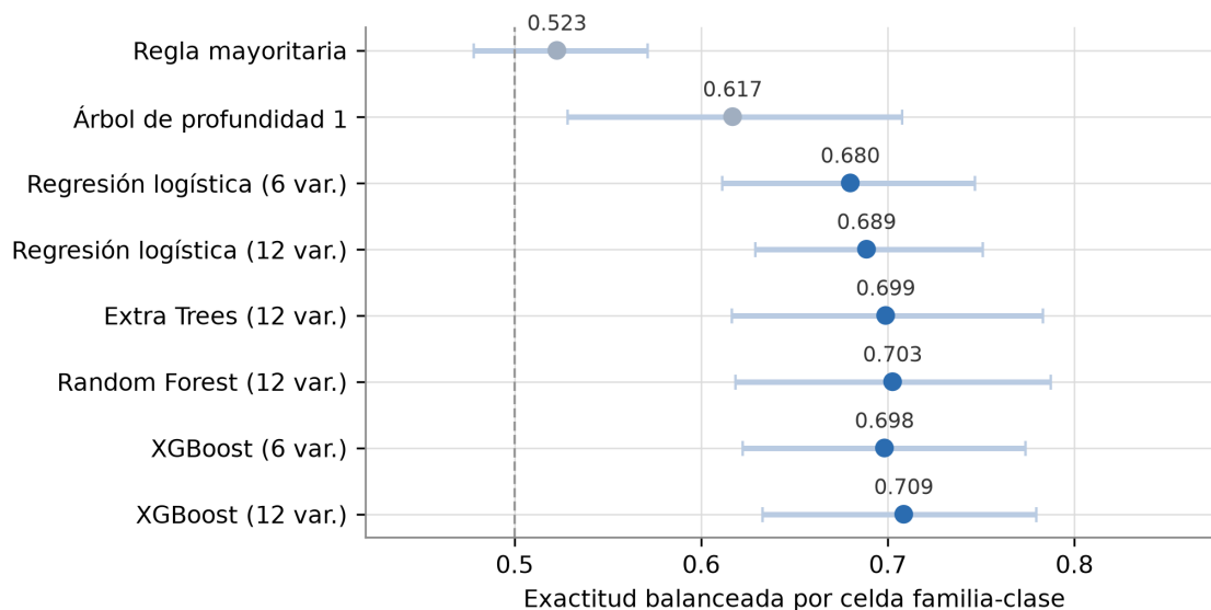
Figura 3.6: Exactitud balanceada por celda de familia y clase de cada modelo, con intervalo de confianza del 95 % obtenido por remuestreo de las 24 familias. Los intervalos se solapan entre todos los modelos con capacidad suficiente. Nota. Elaboración propia.
