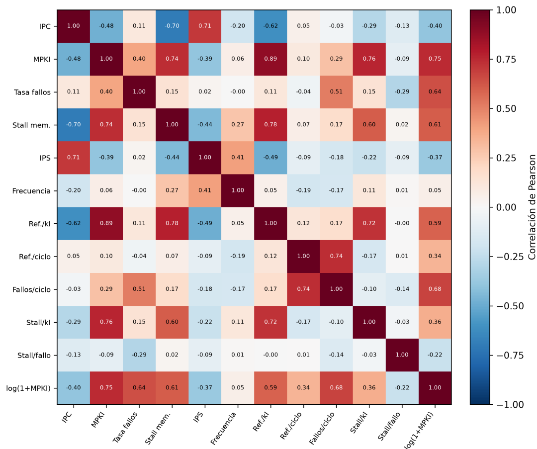
Figura 3.5: Correlación de Pearson entre las 12 variables del candidato congelado sobre la muestra estratificada de 36 310 intervalos. Nota. Elaboración propia.
