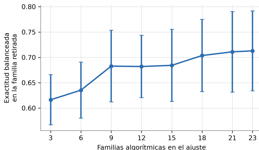
Figura 3.11: Exactitud balanceada sobre la familia retirada en función del número de familias empleadas en el ajuste. Cada punto promedia las 24 familias retiradas y tres repeticiones de la selección; las barras indican el intervalo de confianza del 95 % entre familias. Nota. Elaboración propia.
