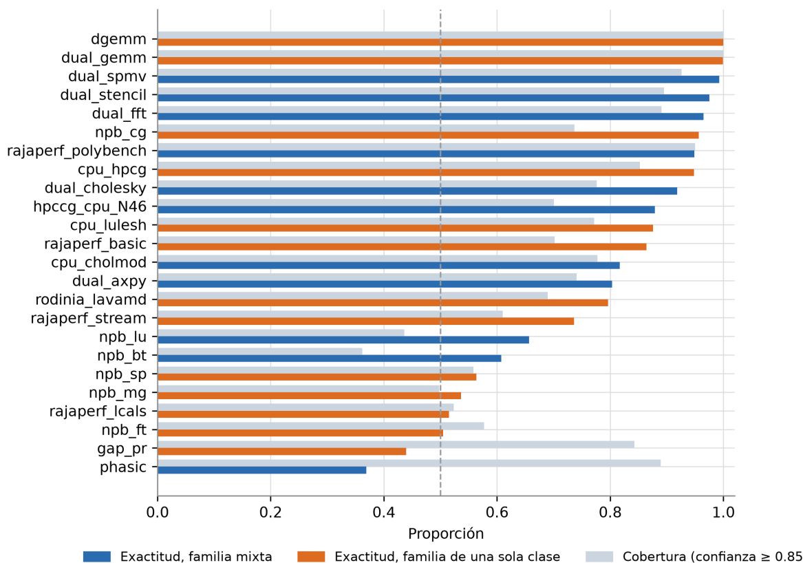
Figura 3.8: Exactitud del modelo final y cobertura de la decisión automática para cada familia retirada. El color distingue las familias que contienen ambas clases de las que contienen una sola. Nota. Elaboración propia.
