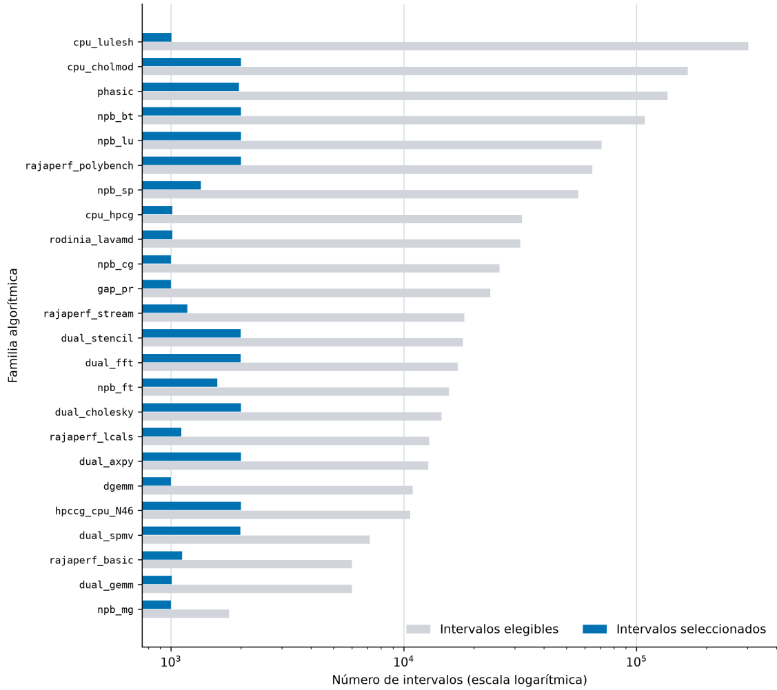
Figura 3.3: Intervalos elegibles y seleccionados por familia algorítmica. El eje logarítmico permite comparar familias cuyo volumen original difiere en varios órdenes de magnitud. Nota. Elaboración propia a partir de family_class_frequency_summary.csv y las predicciones fuera de muestra.
