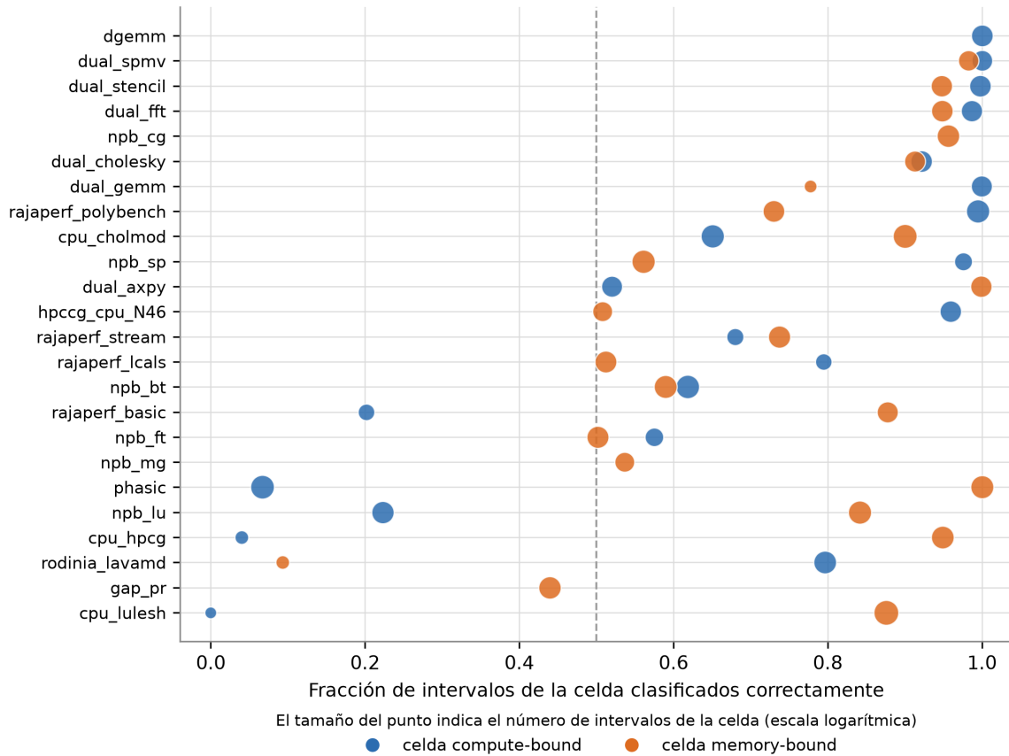
Figura 3.4: Fracción de aciertos del modelo final en cada una de las 44 celdas de familia y clase, con evaluación sobre todos los intervalos de la familia retirada. Las familias con una sola celda son las de una sola clase. Nota. Elaboración propia.
