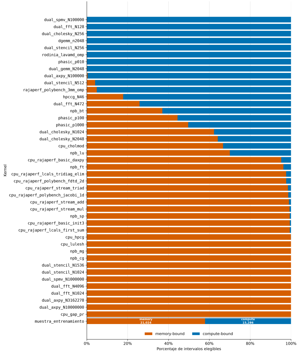
Figura 3.1: Porcentaje de intervalos elegibles clasificados compute_bound y memory_bound para cada configuración de kernel de la campaña CPU. La barra final resume la muestra usada por el clasificador, con 15 286 intervalos compute_bound y 21 024 intervalos memory_bound . Fuente: Elaboración propia.
