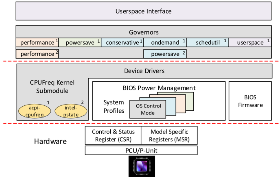
Figura 1.7: Jerarquía de los mecanismos de gestión de rendimiento desde la interfaz de espacio de usuario hasta el hardware. Fuente: tomado de Hebbar y Milenković [25].
