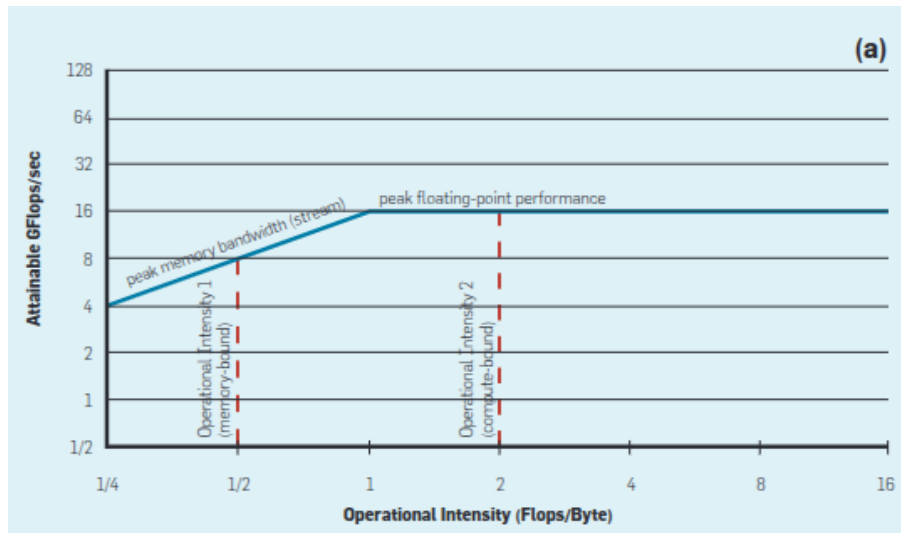
Figura 1.1: Modelo Roofline conceptual y relación entre el techo de ancho de banda de memoria y el techo de rendimiento de cómputo. Tomado de Williams et al. [59, Fig. 1(a)].
