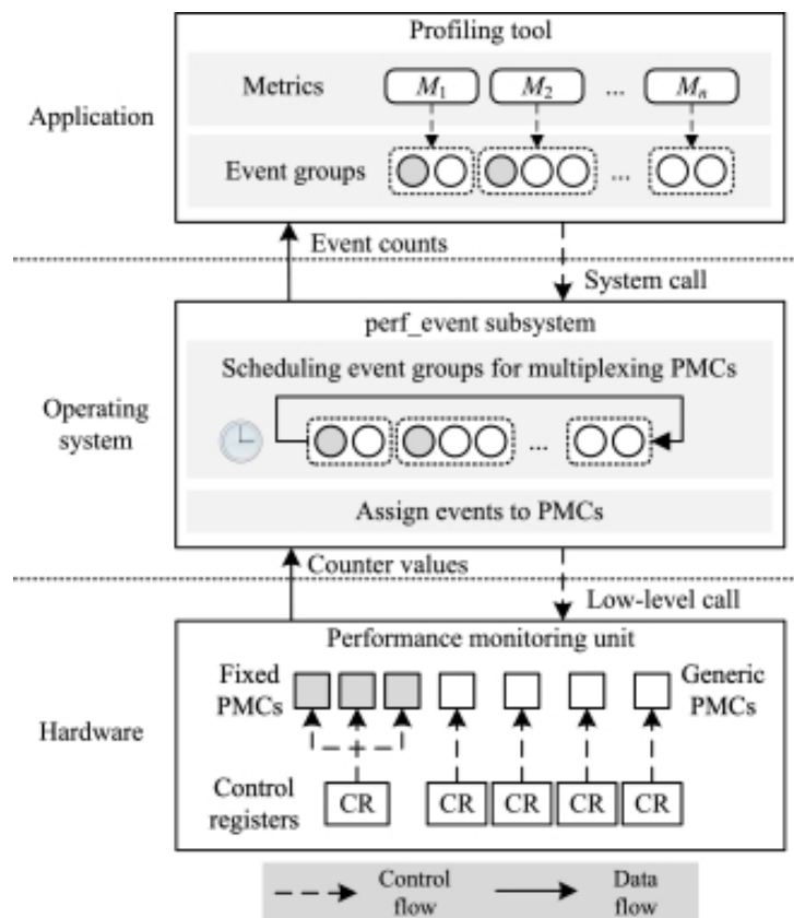
Figura 1.4: Flujo de configuración y lectura de eventos de rendimiento mediante el subsistema perf_event de Linux. Fuente: tomado de Liu et al. [42].
