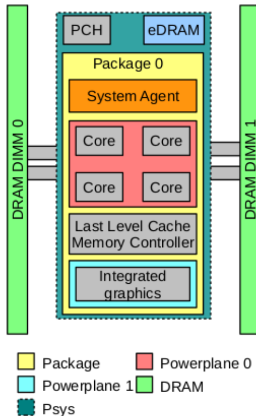
Figura 1.5: Dominios energéticos expuestos mediante Intel RAPL. Fuente: tomado de Thamm y Leser [53].
