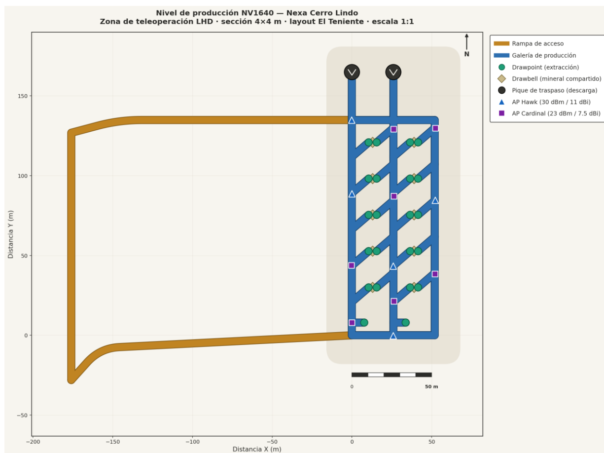
Figura 9. Geometría real de la zona de producción y ubicación de los AP en ns-3 NS-3.
