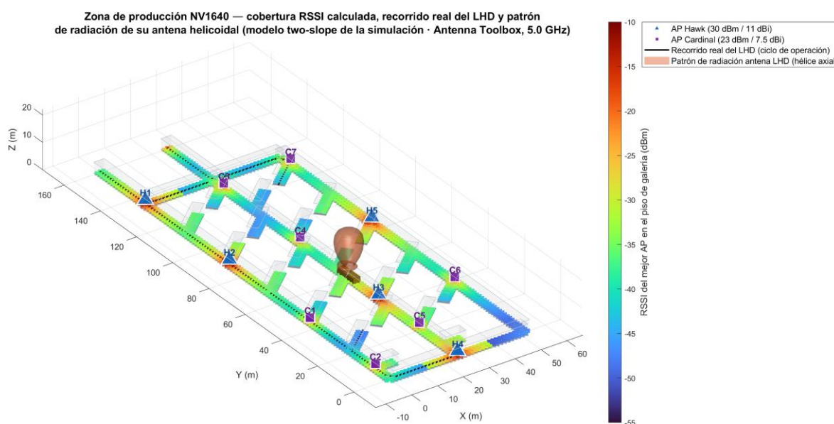
Figura 9. Entorno tridimensional de la zona de producción: cobertura RSSI calculada, recorrido real del LHD, los 12 AP y patrón de radiación de la antena del vehículo.
