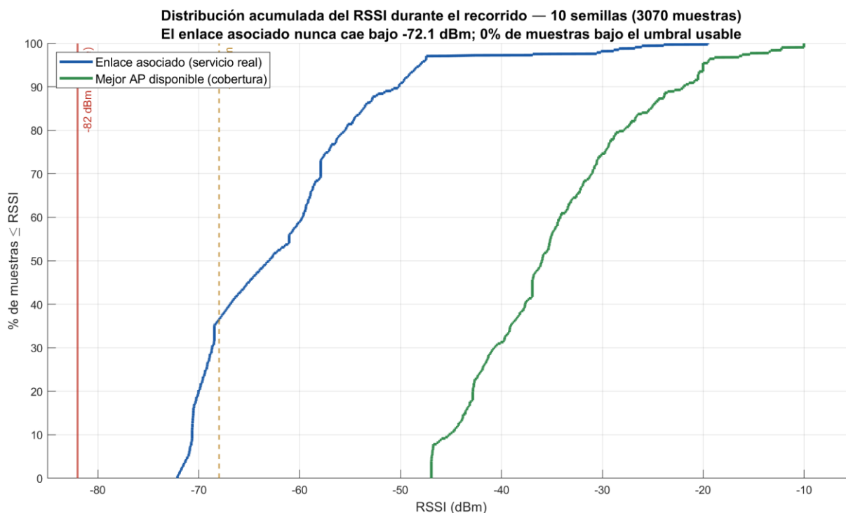
Figura 21. Distribución acumulada del RSSI del enlace asociado y del mejor AP durante el recorrido (diez semillas).
