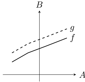
Rysunek 11: Porządek pionowy f \sqsubseteq g \iff \forall a \in A \quad f(a) \sqsubseteq_B g(a) . Wykres funkcji g (linia przerywana) leży nad wykresem funkcji f (linia ciągła).
