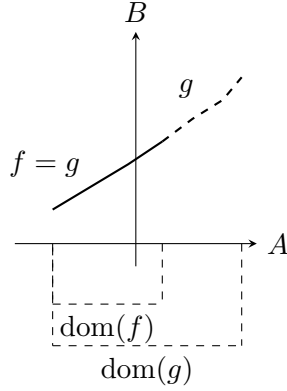
Rysunek 10: Porządek poziomy f \sqsubseteq g \iff f \subseteq g . Funkcja g (linia ciągła i przerywana) rozszerza f (linia ciągła), tzn. pokrywa się z f na \text{dom}(f) \subseteq \text{dom}(g) i jest dodatkowo określona poza \text{dom}(f) .
