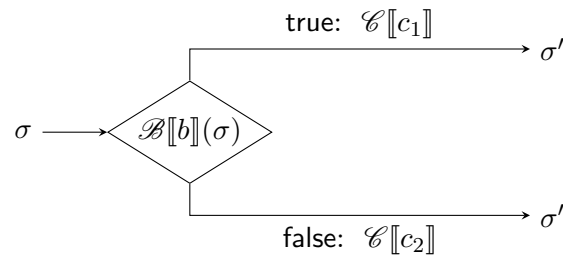
Rysunek 6: Denotacja instrukcji warunkowej: wartość warunku b w stanie \sigma decyduje, czy stan końcowy wyznacza denotacja c_1 , czy c_2 .
