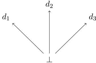
Rysunek 8: Porządek płaski na zbiorze D_\perp = \{\perp, d_1, d_2, d_3\} .
