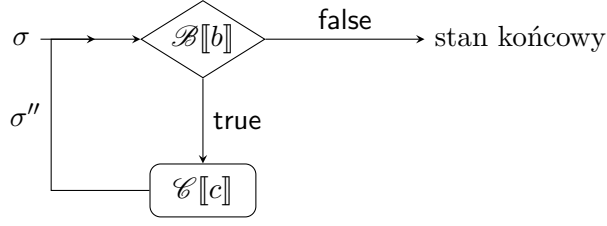
Rysunek 7: Wykonanie pętli while b do c : po każdym wykonaniu ciała c wracamy do sprawdzenia warunku b w nowym stanie \sigma'' .
