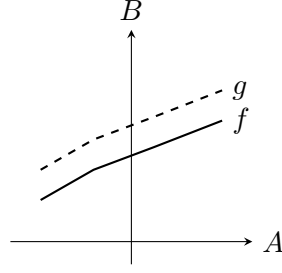
Rysunek 10: Porządek pionowy: f \subseteq g \iff \forall a \in A \ f(a) \subseteq_B g(a) . Wykres funkcji g (linia przerywana) leży nad wykresem funkcji f (linia ciągła).
