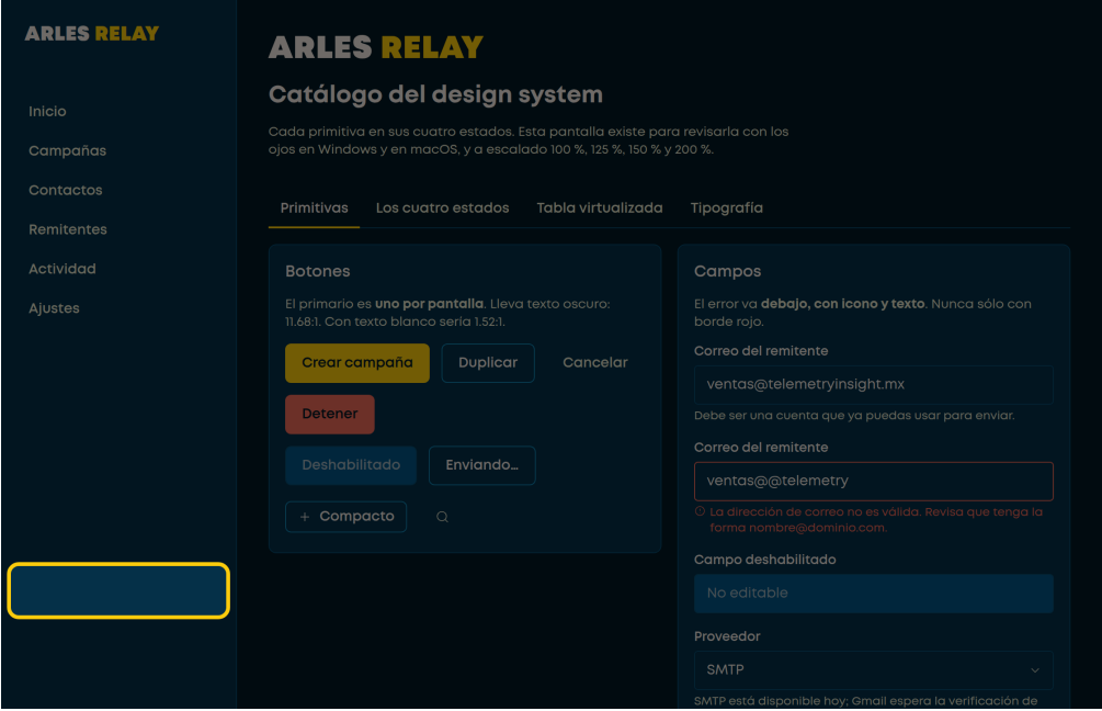
Referencia · Primitivas
