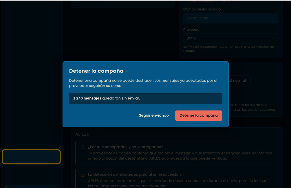
Referencia · Modal
