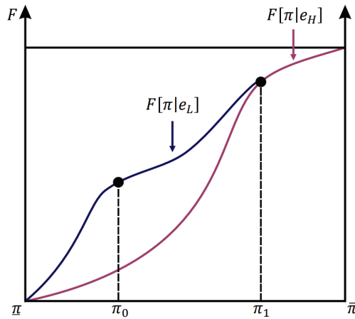
Figura 39: Funciones de distribución.
