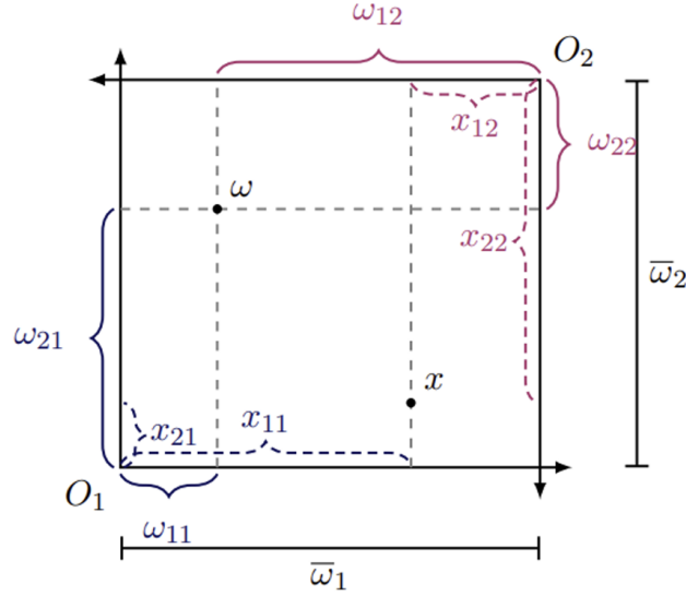
Figura 1: Caja de Edgeworth
