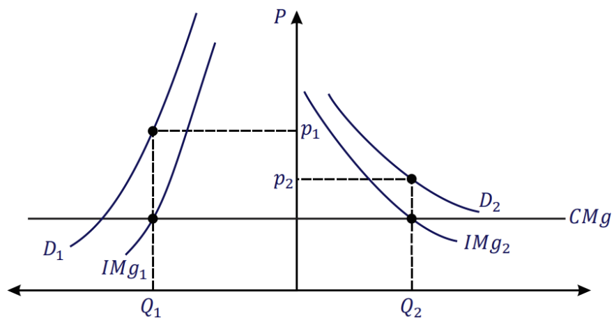
Figura 28: Discriminación de tercer grado.
