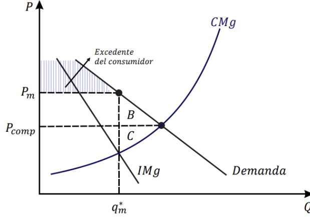
Figura 24: Maximización de beneficios
