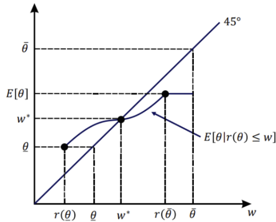
Figura 34: Equilibrio competitivo bajo selección adversa.
