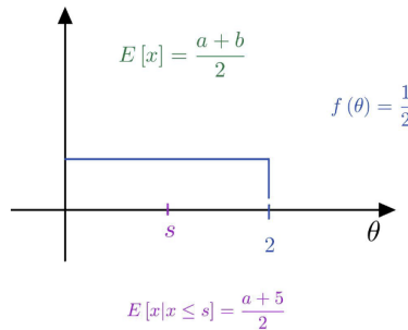
Figura 36: Gráfico de densidad.
