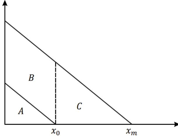
Figura 27: Discriminación de segundo grado.
