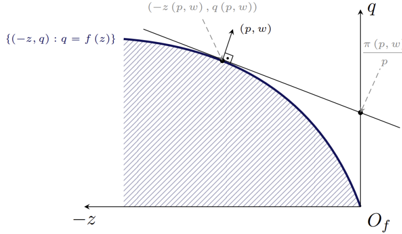
Figura 17: Problema de la firma
