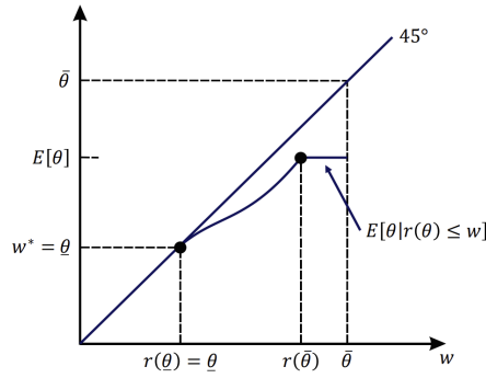
Figura 35: Equilibrio competitivo bajo selección adversa.
