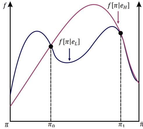
Figura 38: Funciones de densidad.
