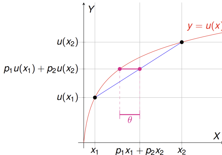
Figura 33: Prima de aversión al riesgo
