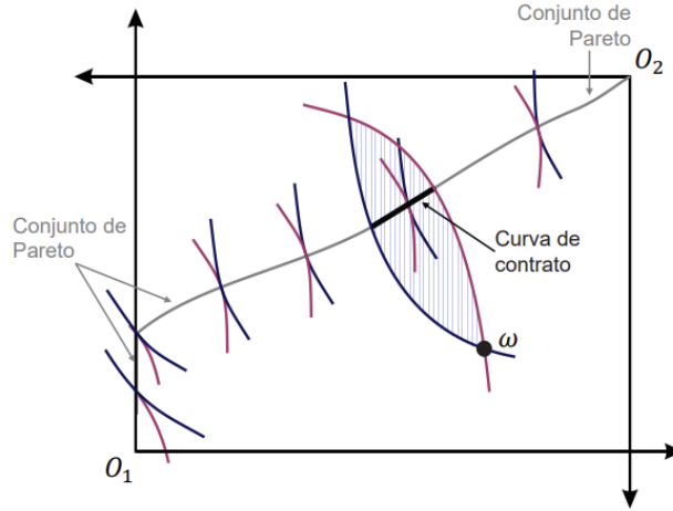
Figura 15: Conjunto de Pareto y Curva de Contrato
