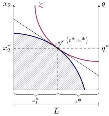
Figura 19: Equilibrio en el modelo de Robinson Crusoe
