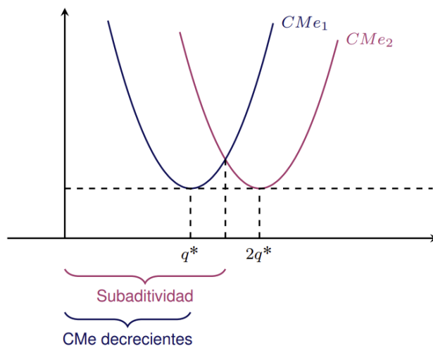
Figura 20: Subaditividad de costos
