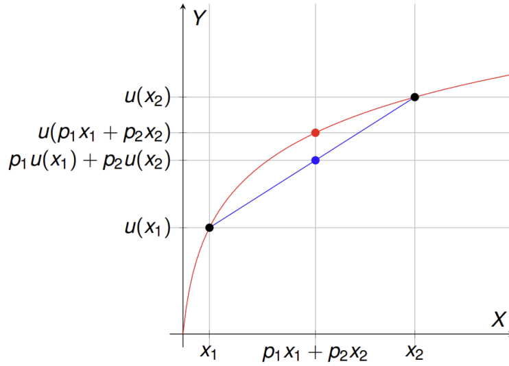
Figura 32: Aversión al riesgo
