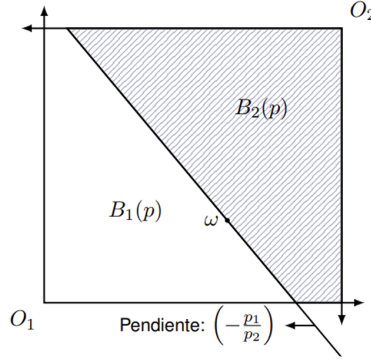
Figura 2: Conjunto presupuestario B_i(p)
