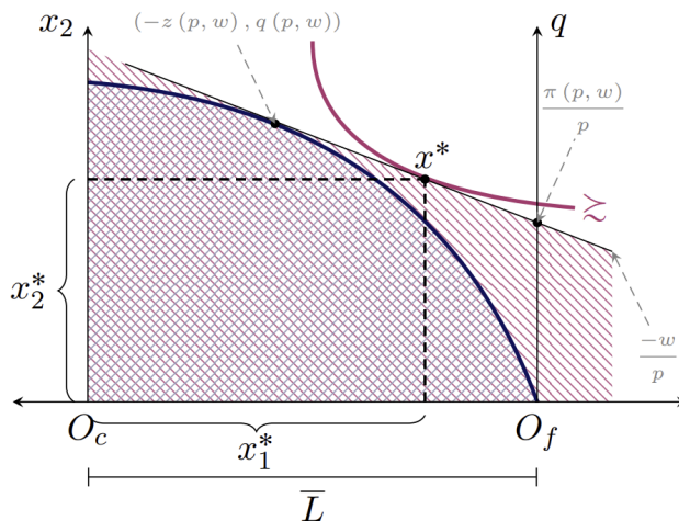
Figura 18: Problema del consumidor
