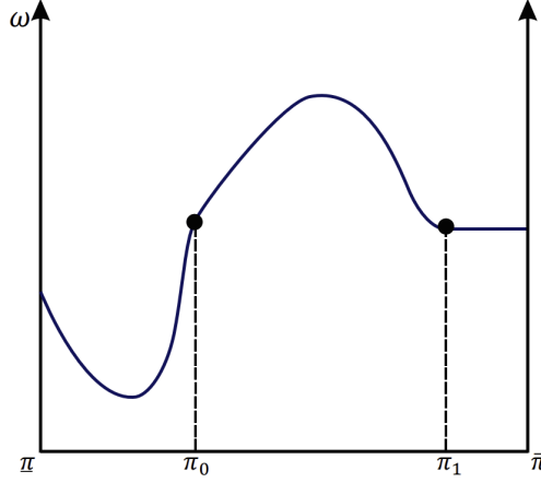
Figura 40: Esquema óptimo de pagos.
