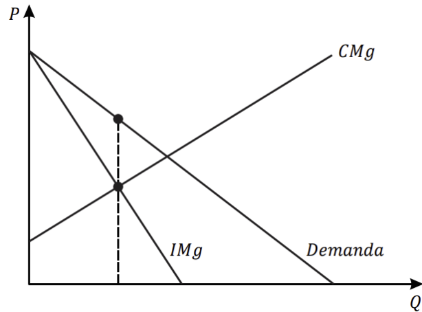
Figura 22: Maximización de beneficios
