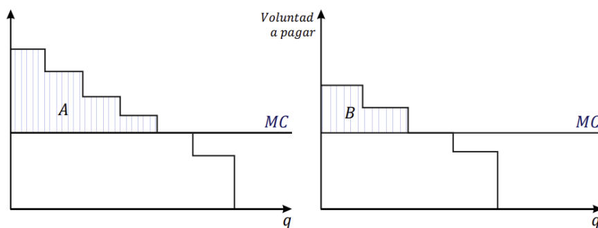
Figura 25: Voluntad a pagar.
