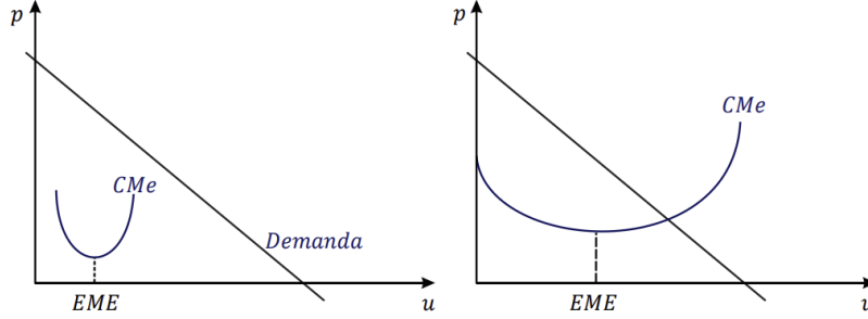
Figura 21: Escala mínima eficiente (EME)
