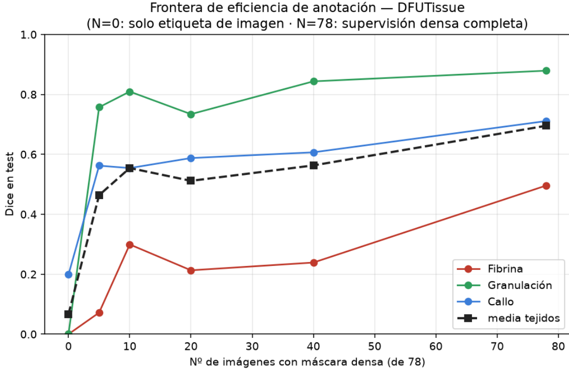
Figura 1.4: Frontera de eficiencia de anotación en DFUTissue (resultado preliminar, una semilla).
