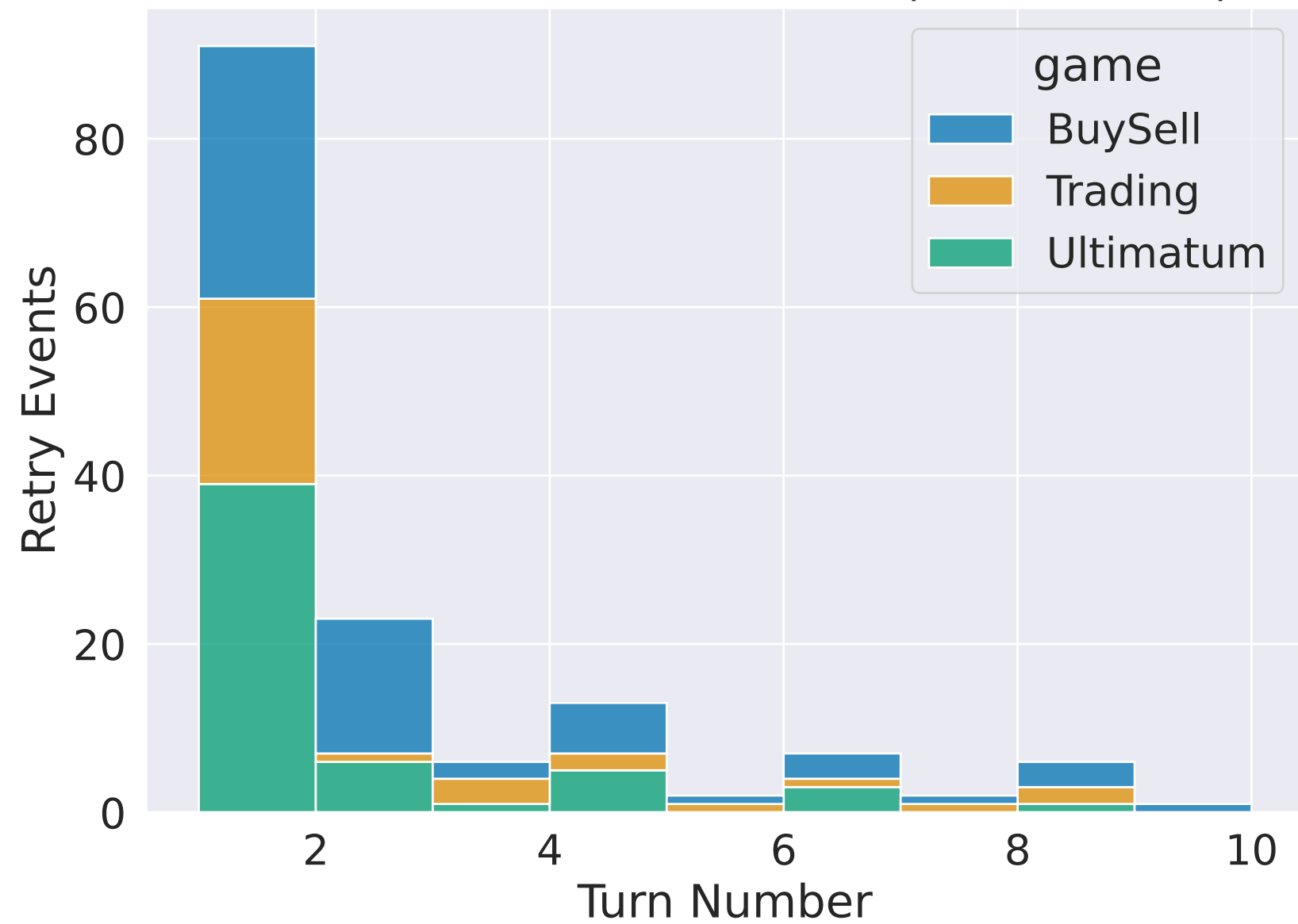
When Do Parse Errors Occur? (Turn Number)
