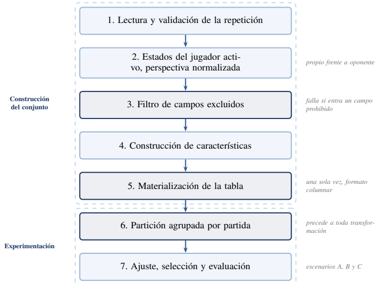
Figura 5. Tuber a propuesta. Las etapas 1 a 5 se ejecutan una sola vez y producen la tabla; las etapas 6 y 7 operan sobre ella. El filtro de campos excluidos y la partici n agrupada se imponen mediante pruebas autom ticas y no por convenci n.
