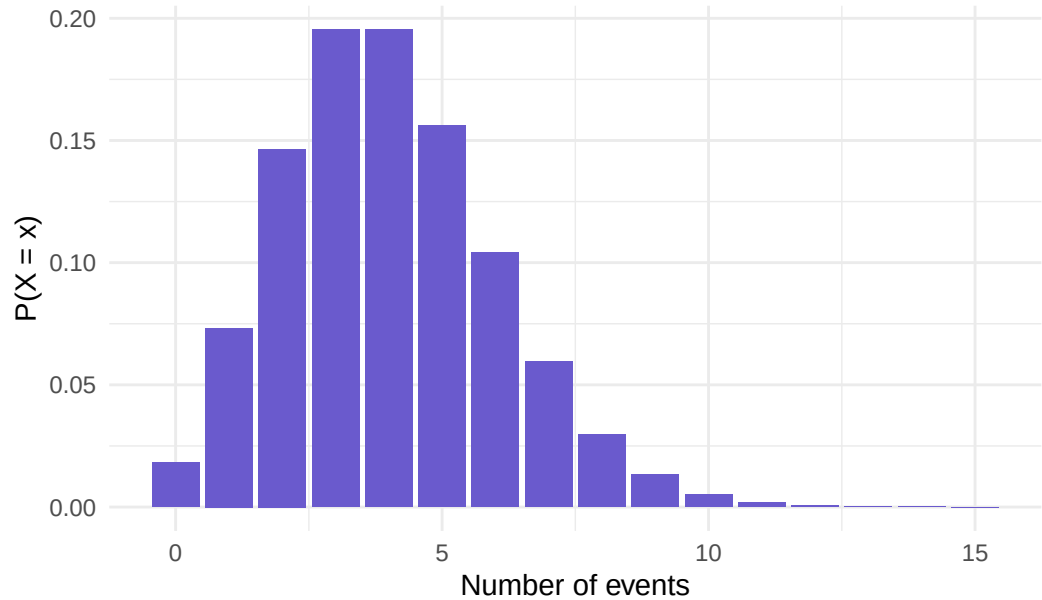
Poisson( \lambda = 4 )
