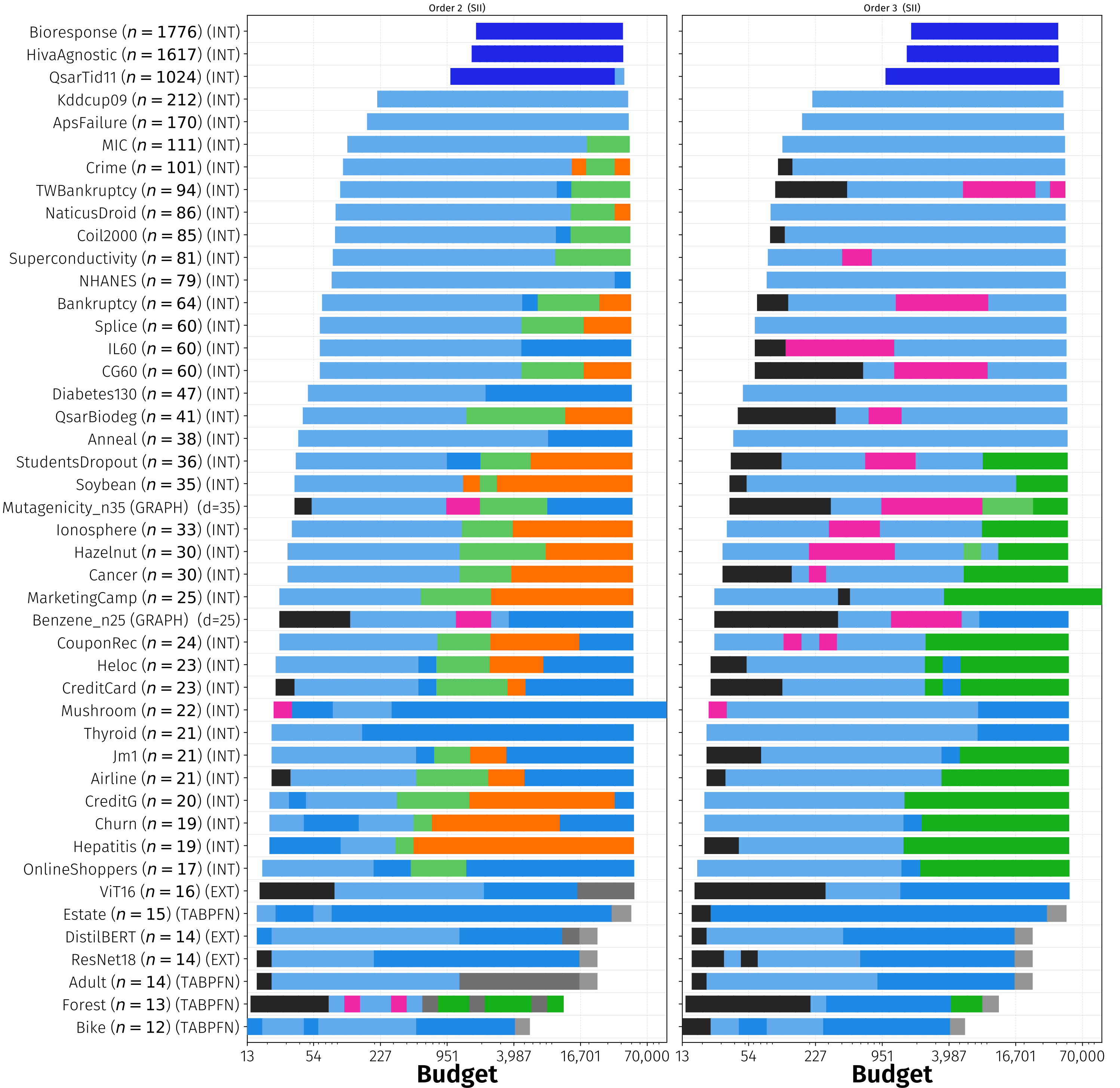
Dataset
