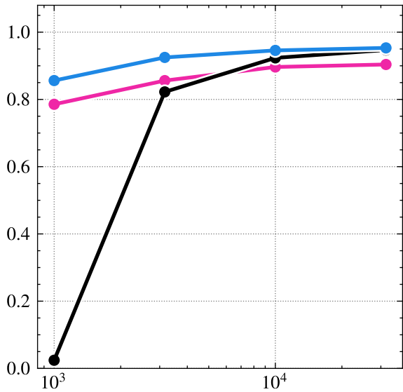
FIxLIP: ViT32
