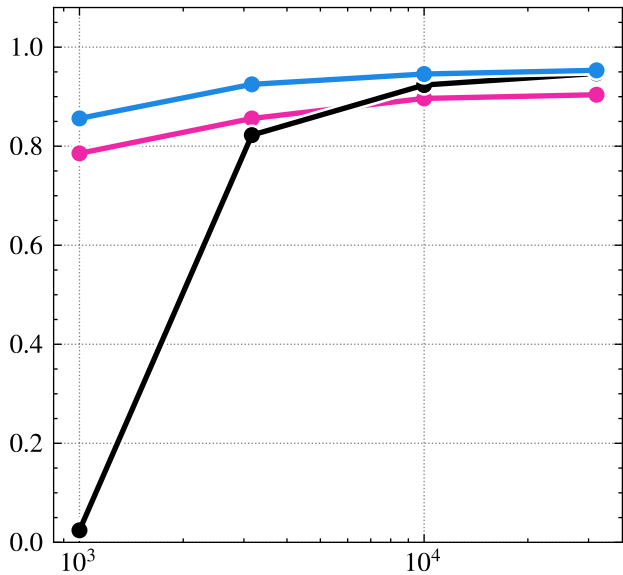
FIxLIP: ViT32
