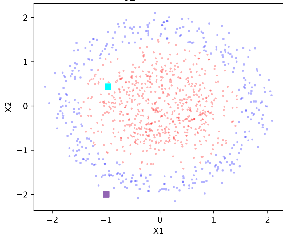
ring_dataset - Face
