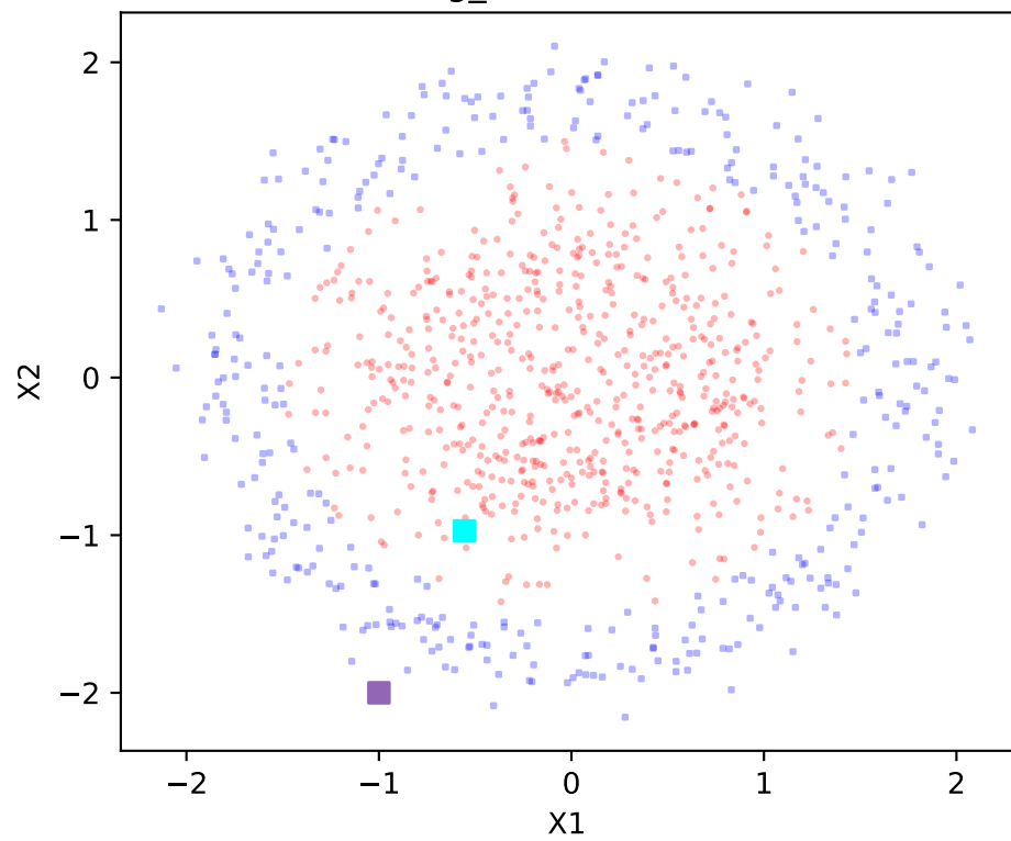
ring_dataset - Face
