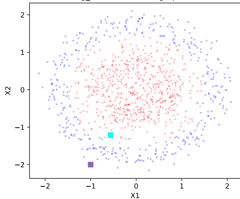
ring_dataset - DICE
