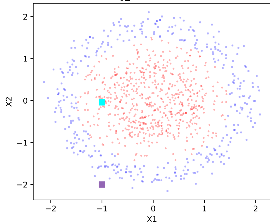
ring_dataset - DICE
