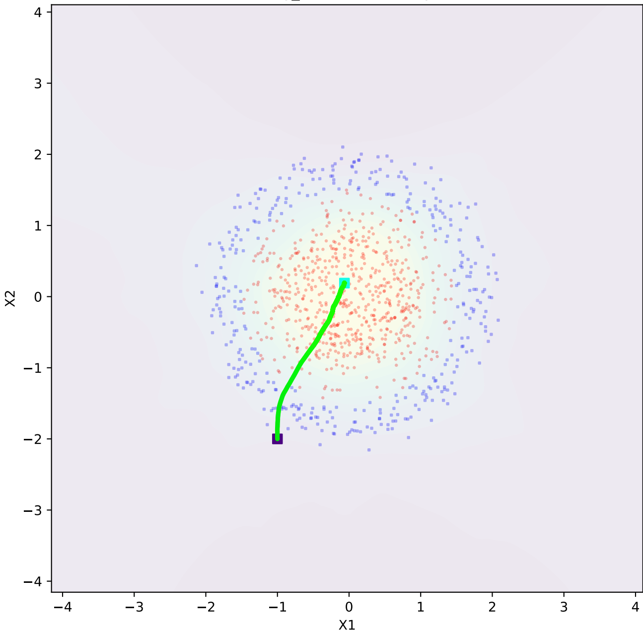
ring_dataset - validity
