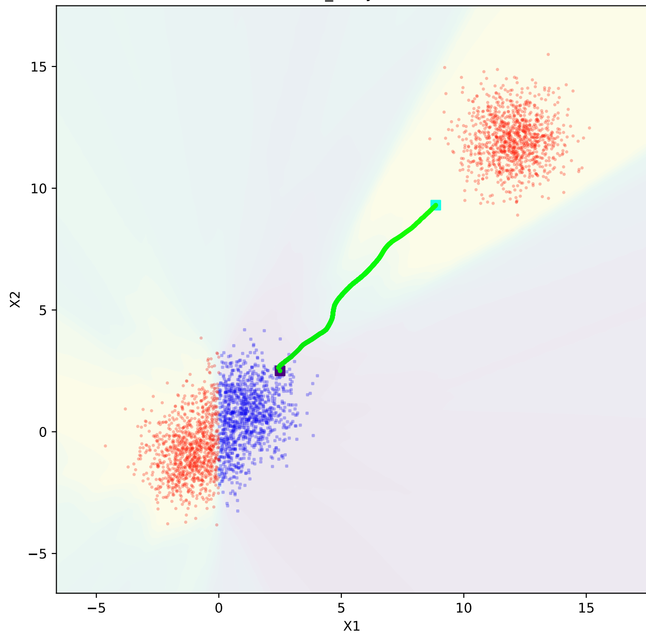
bubbles_noisy - robust
