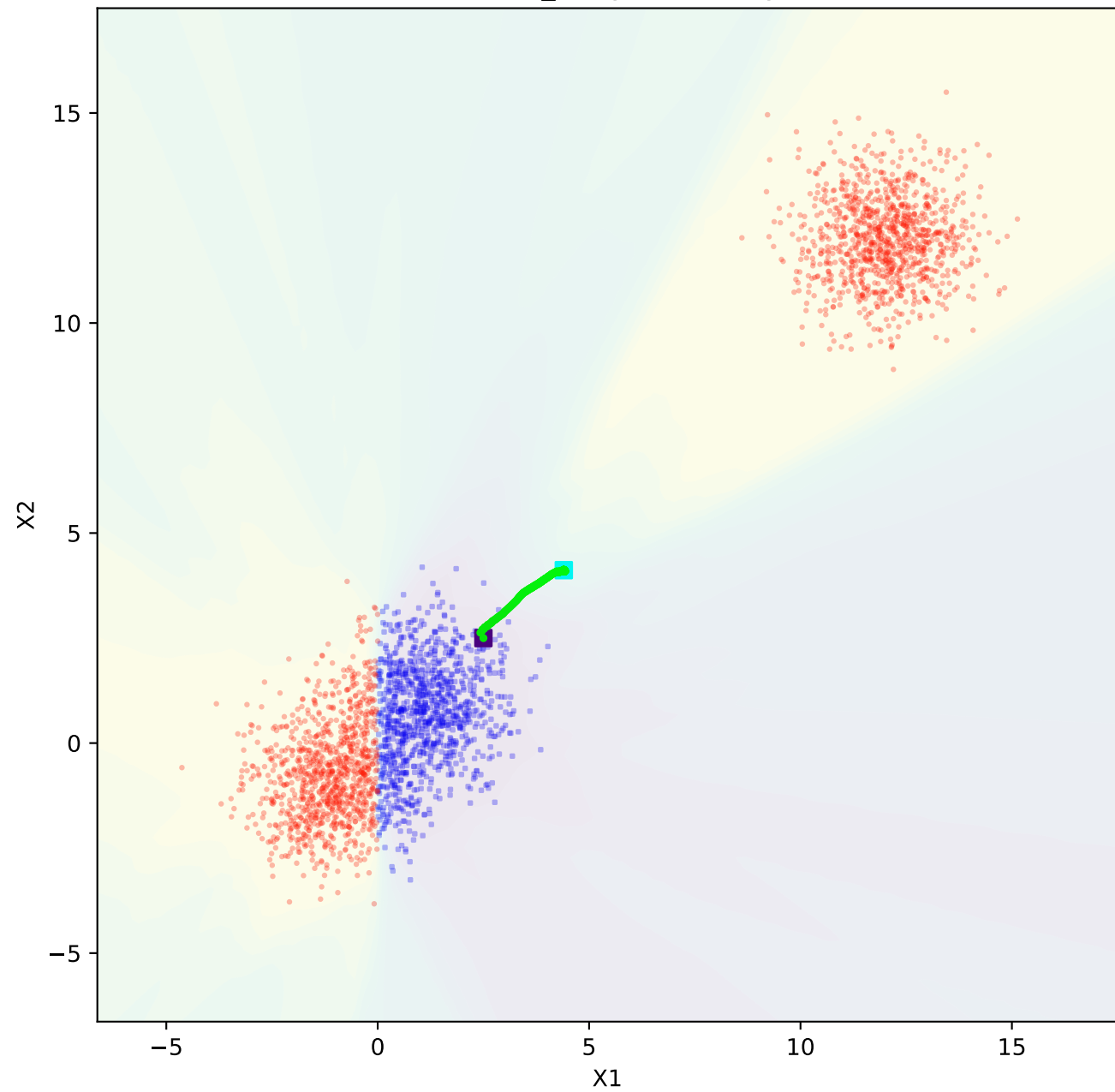
bubbles_noisy - similarity
