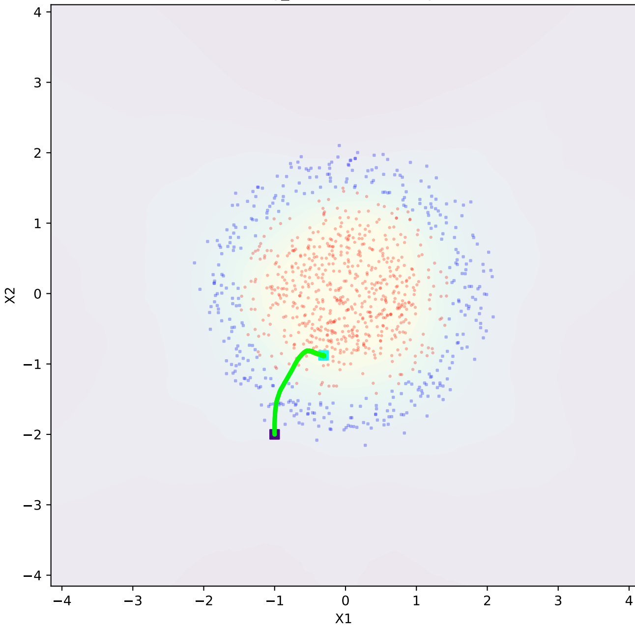
ring_dataset - similarity
