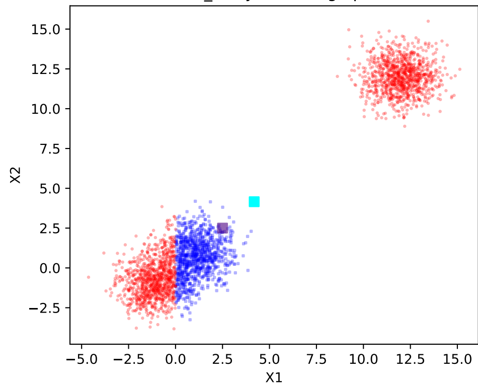
bubbles_noisy - DICE
