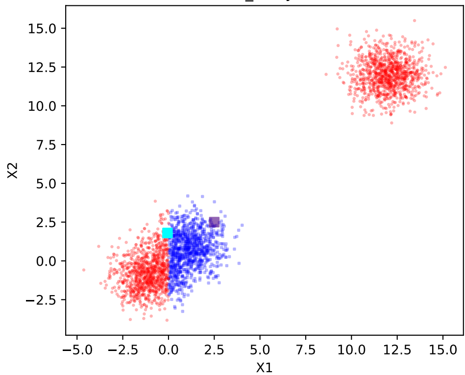
bubbles_noisy - Face
