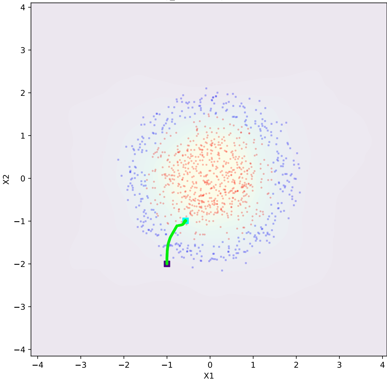
ring_dataset - plausible
