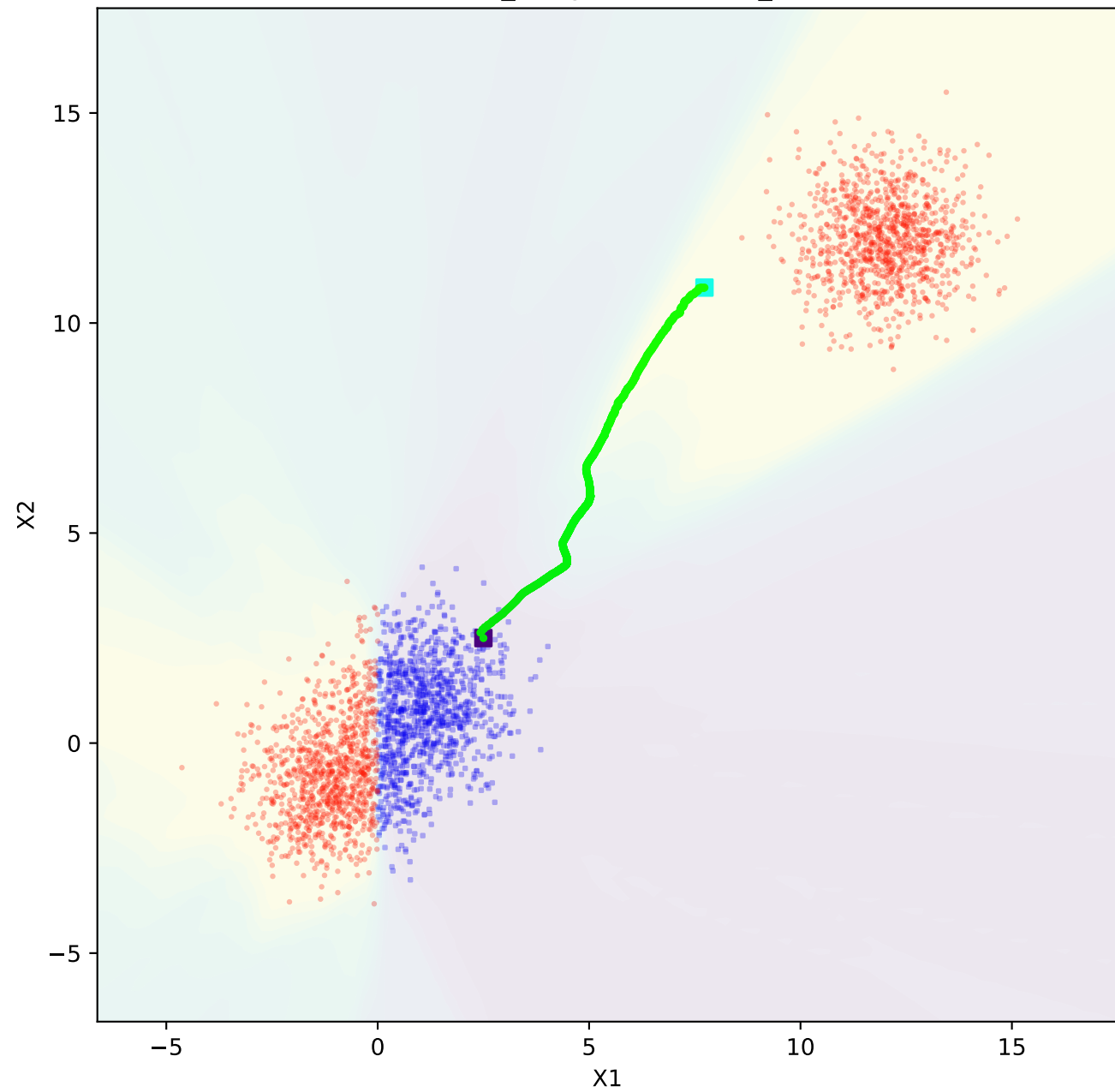
bubbles_noisy - connected_ball
