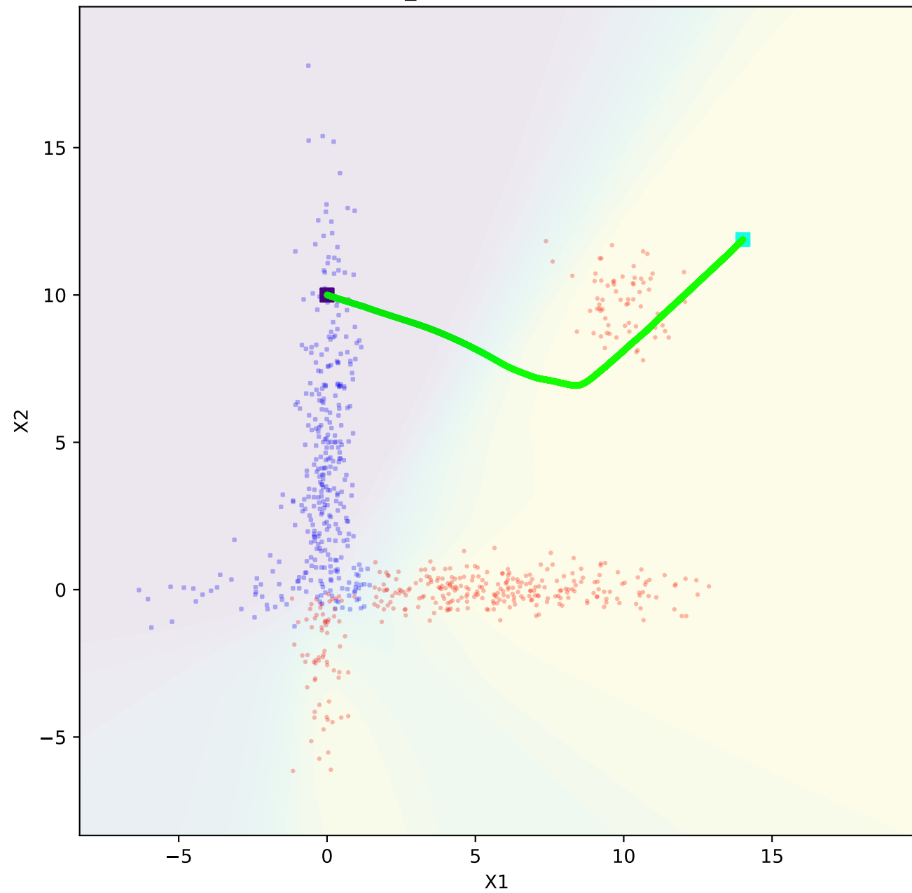
l_dataset - robust
