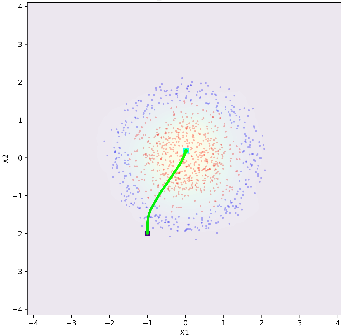
ring_dataset - robust
