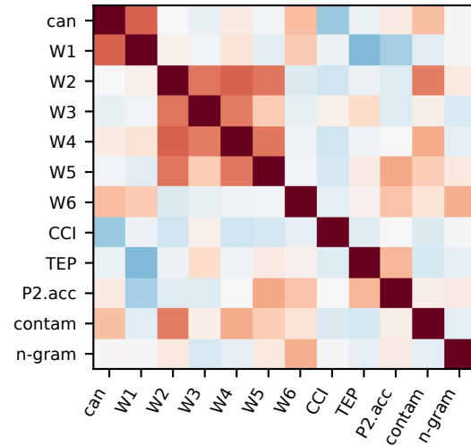
GPT-4o
