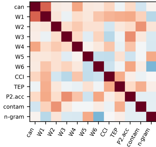
Llama
