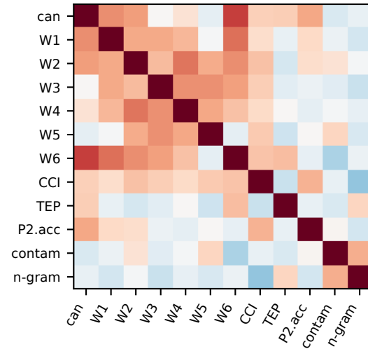
Gemini
