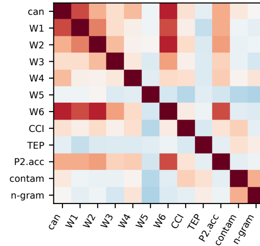
Claude
