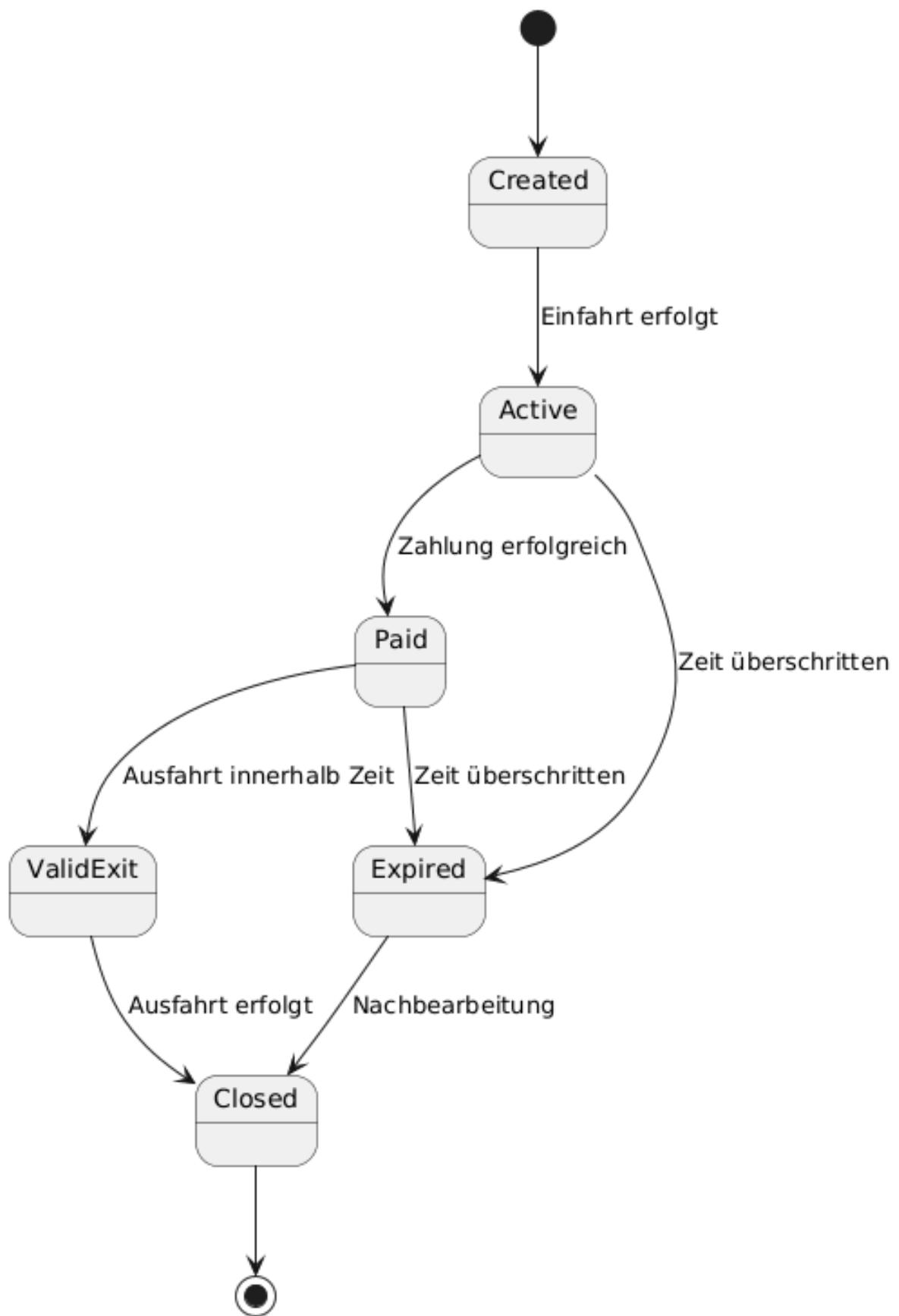
Abbildung 11: Ticket Zustandsdiagramm
