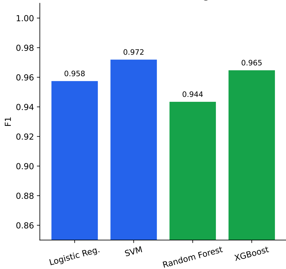
RQ4: F1 at 20% Data Degradation
