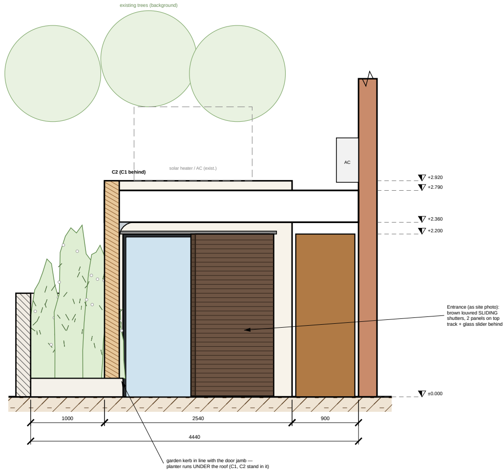
2/V1-02 PLANTS-SIDE ELEVATION — C1 + C2 — 1:50
