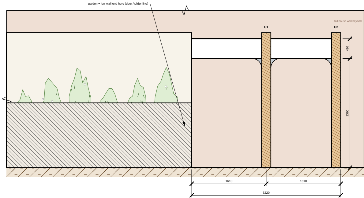
2/V1-02 PLANTS-SIDE ELEVATION — C1 + C2 — 1:50
