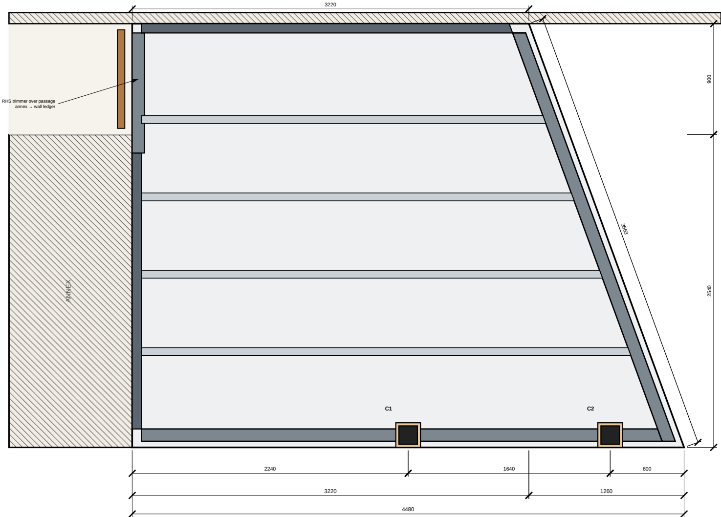
2/V1T-01 ROOF FRAMING PLAN — 1:30
