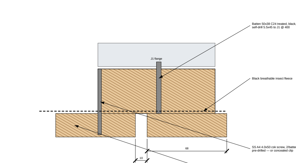
D6 SOFFIT SLAT FIXING — 1:2
