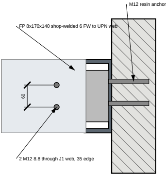
C1 J1 -- LEDGER L1 — 1:10
