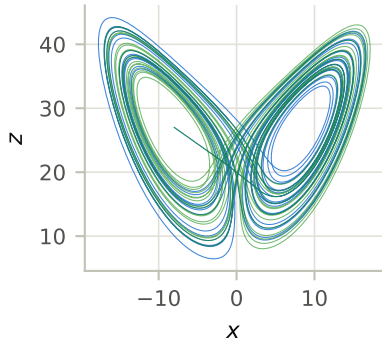
Lorenz
