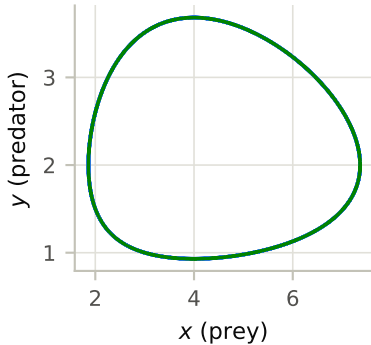
Lotka-Volterra
